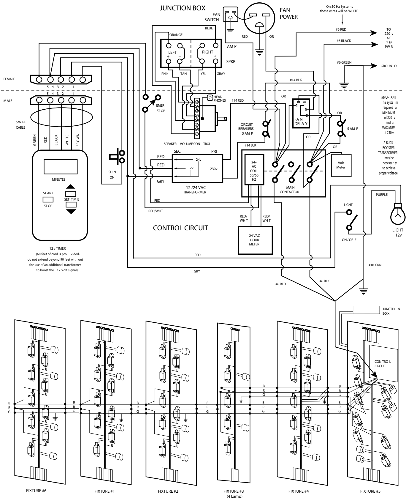
S I N G L E P H A S E S Y S T E M S C H E M A T I C
