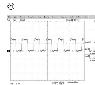
CN401 PIN13:AOUT_MCLKOUT
