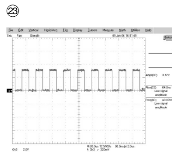
CN400 PIN28:AOUT_FSYNC
