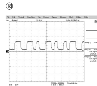
CN400 PIN1:AOUT_ICE958
