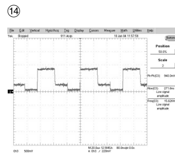
CN400 PIN10:VOUT_G/Y
