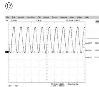
CN901 PIN108:27MHZ
