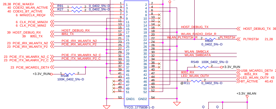
Mini WLAN
