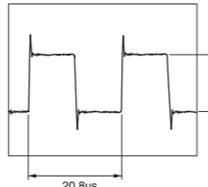
(WF06) PCMF3 (SD-7:E4)
