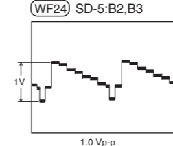
Component Y waveform (WF24) SD-5:B2,B3
