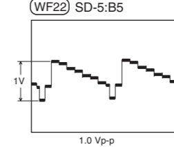
S-Video Y waveform (WF22) SD-5:B5
