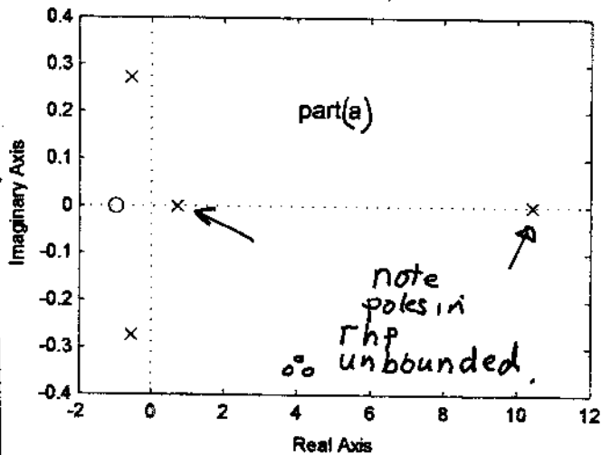
Pole-Zero Map
