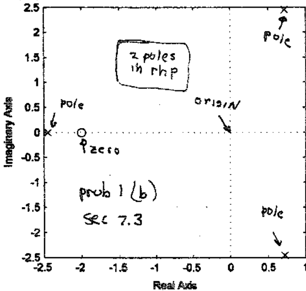
Pole-Zero Map
