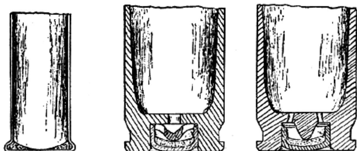
SEPARATE ANVIL PRIMER "BERDAN" PRIMER
