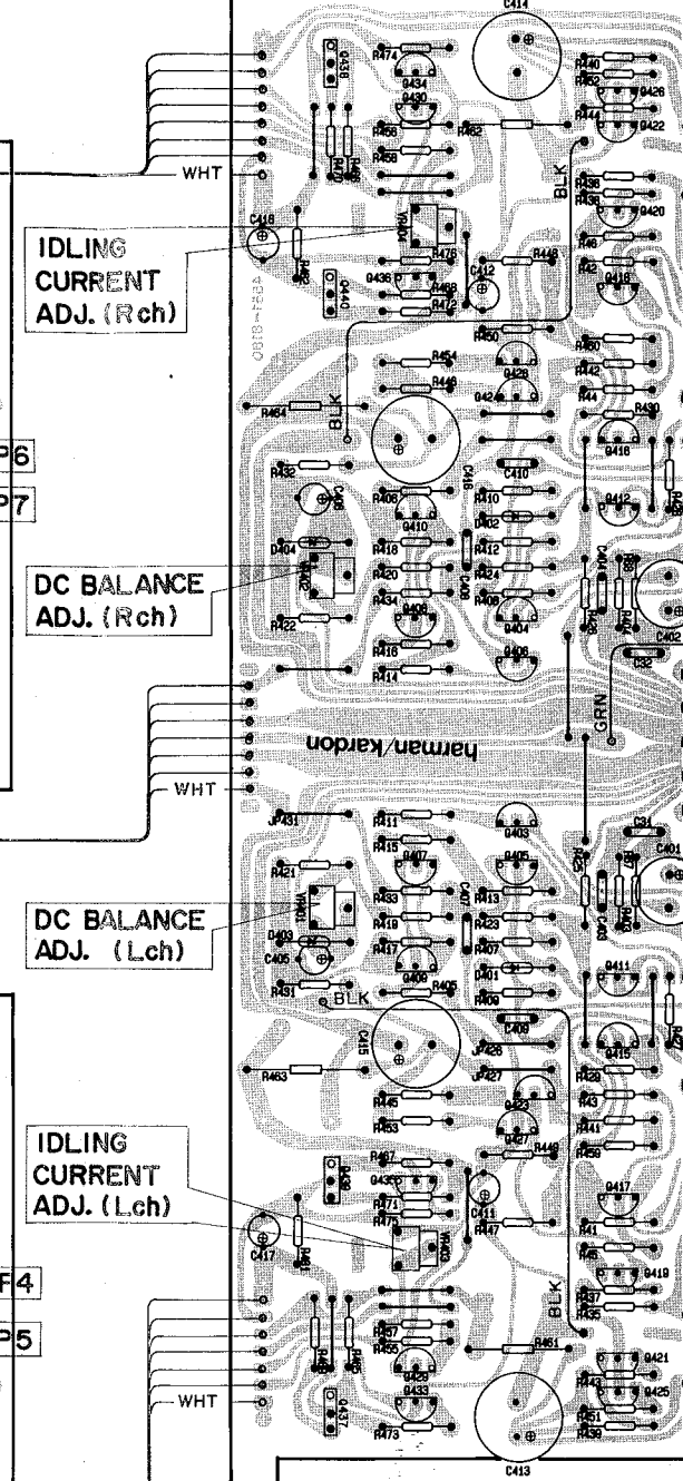
PCB-3
