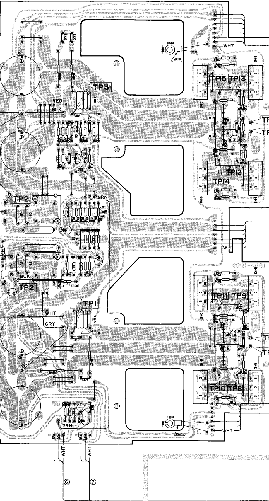
PCB-1
