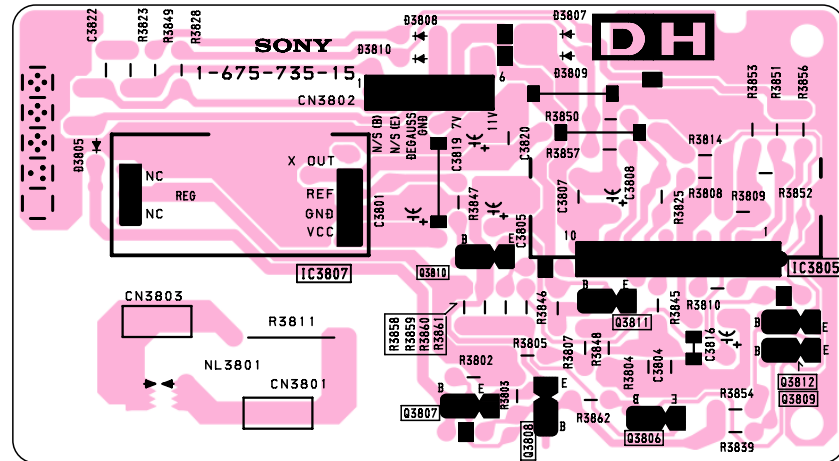
– DH Board –
