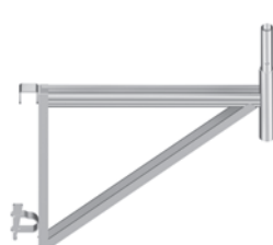
► Ménsula para vanos intermedios, de 0,73 m.
