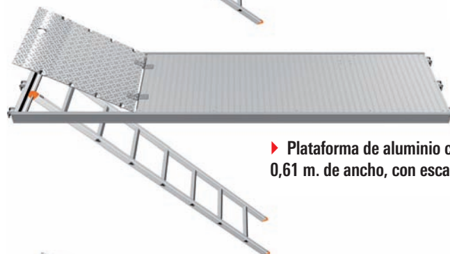
▶ Plataforma Robust T9 con enganche a tubo redondo con trampilla, de 0,61 m. de ancho, con escalerilla integrada
