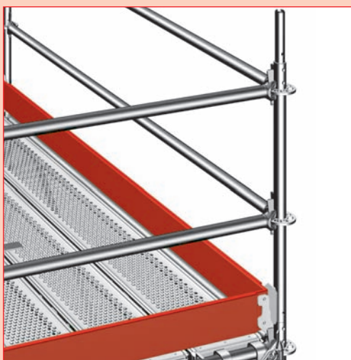
▶ Rodapié Allround de acero para tubo
