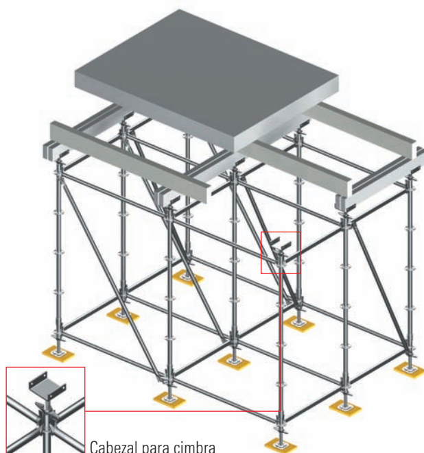
Cabezal para cimbra
