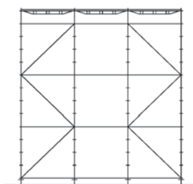
Sección A-A
