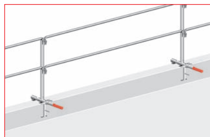
Ejemplo de aplicación de la mordaza para forjado en petos
