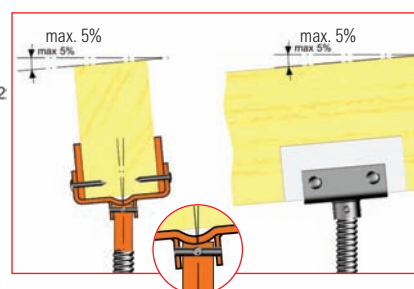
► Cabezal de cimbra 45/60, de inclinación variable macizo de 16 cm.
