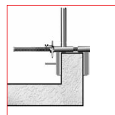
Instalación en peto
