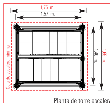
Planta de torre escalera
