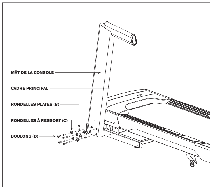
RONDELLE PLATE (B) 8 mm Qté : 8
