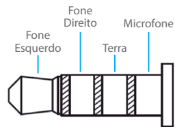
Fone de ouvido com microfone integrado (conector padrão CTIA)
