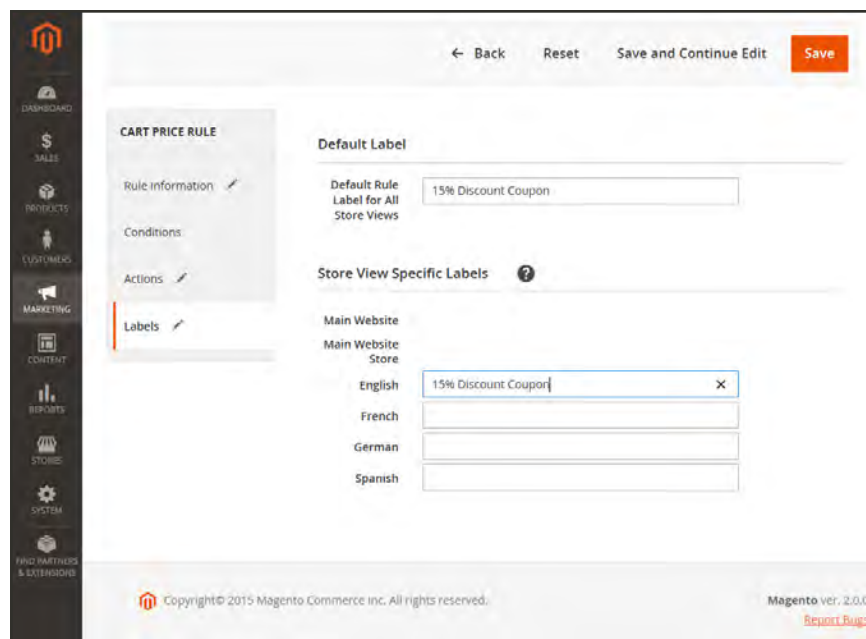
Default Label
