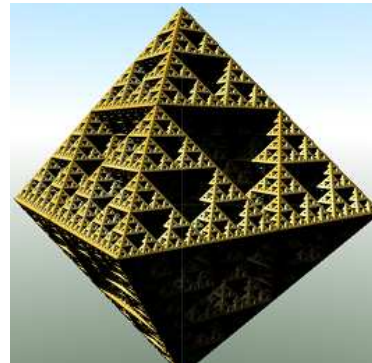
Figure 2.3: Sierpinski
