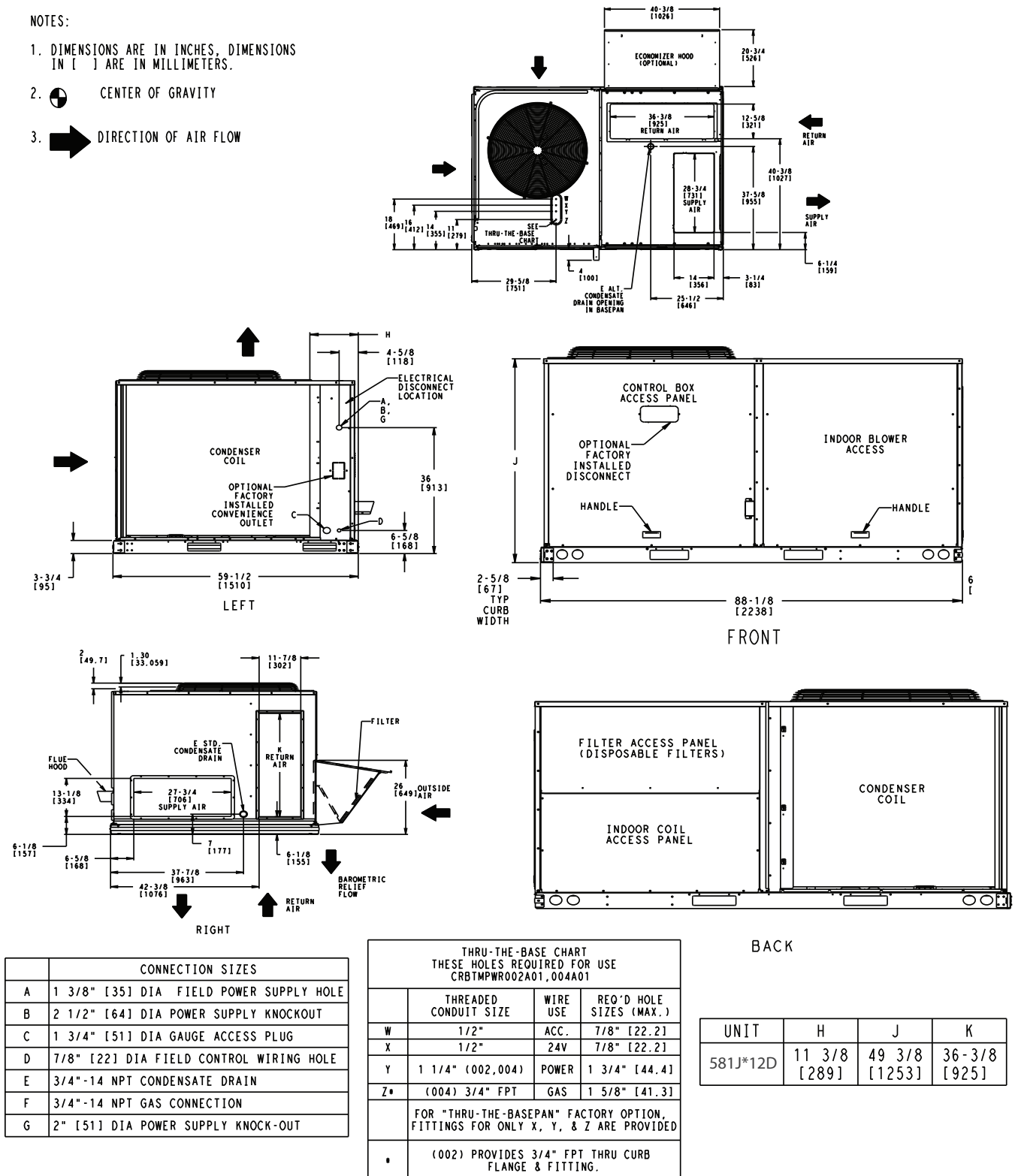
Fig. 9 - Dimensions 581J 12
