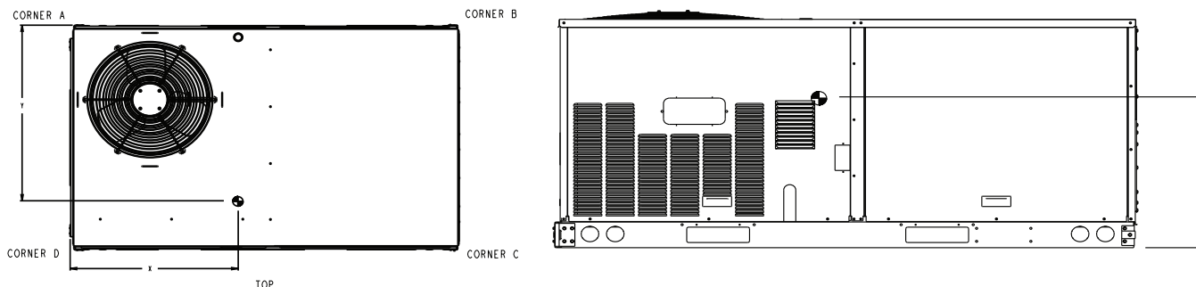
Fig. 2 - Dimensions 581J 04-06
