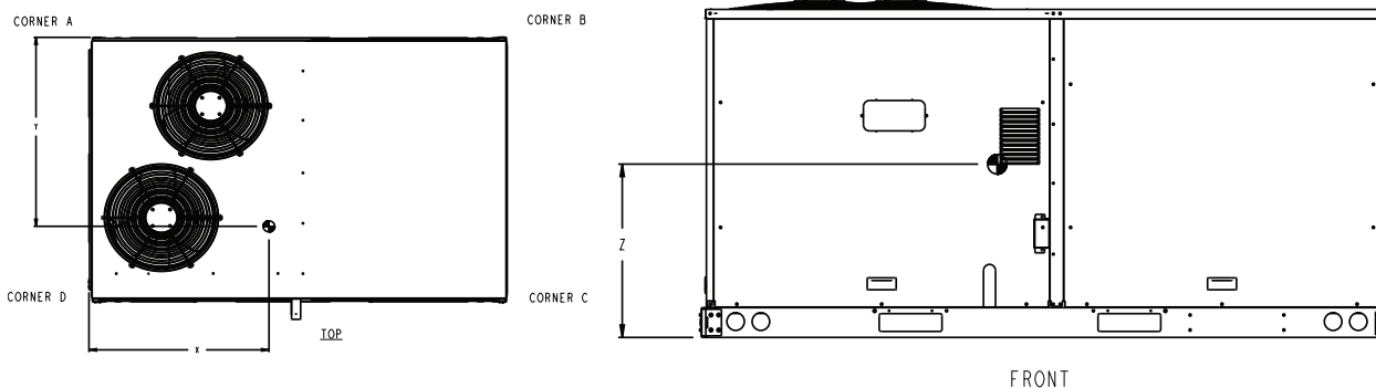
Fig. 6 - Dimensions 581J 07-09
