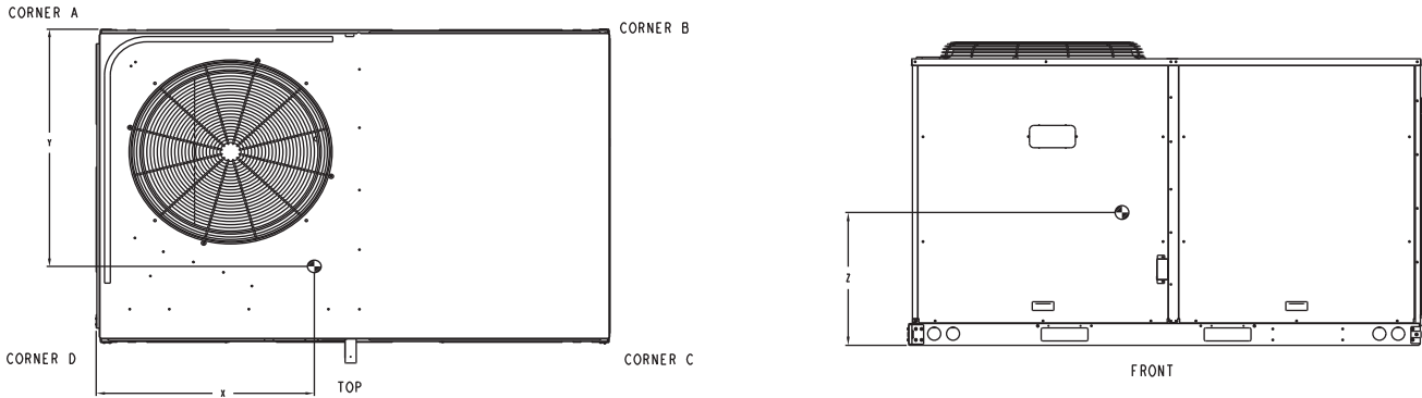
Fig. 10 - Dimensions 581J 12
