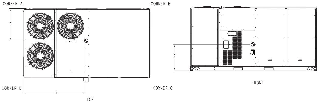
Fig. 14 - Dimensions 581J 14
