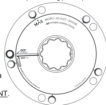
Figura 2: Alinee el centro del agujero del plato Q-Ring, marcado con los puntos de regulación OCP, con la flecha de referencia " OCP+1/2 ", girando ligeramente el plato Q-Ring sobre la araña en sentido anti-horario. Para el caso del plato interior, gire el plato Q-Ring sobre la araña en sentido horario. Si se elige una posición " OCP+1/2 " en el plato Q-Ring exterior, su plato interior Q-Ring debe de estar posicionado igualmente en posición " OCP+1/2 ". Sitúe los tornillos del plato en la posiciones marcadas como ALTERNATIVE BOLT PLACEMENT .
