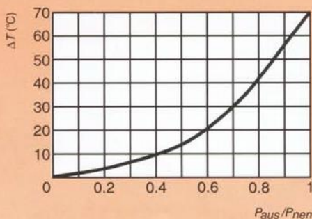
Typische Anwärmung in Abhängigkeit von Belastungsverhältnis P_{aus}/P_{nen}
