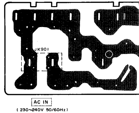
G AC IN/AC OUTLET P.C.B. For[G]AREAS.
