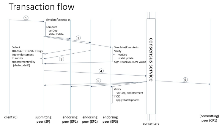
图 1.14.2.2 - 示例交易过程
