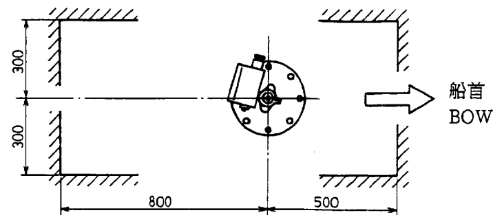
推奨保守点検用スペース (尺度 1/20) RECOMMENDED SERVICE SPACE (SCALE 1/20)
