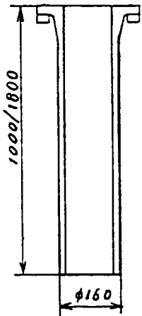
FRP製格納タンク外觀図 FRP RETRACTION TANK OUTLINE DRAWING
