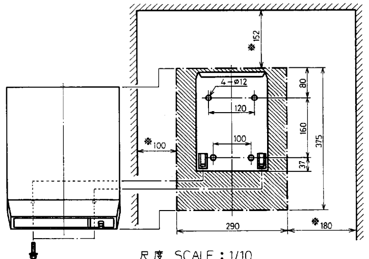
取付寸法 MOUNTING DIMENSION
