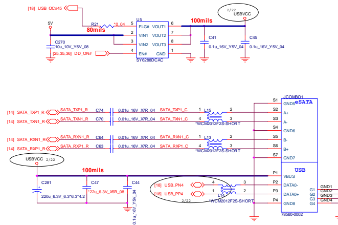
ESATA+USB & POW
