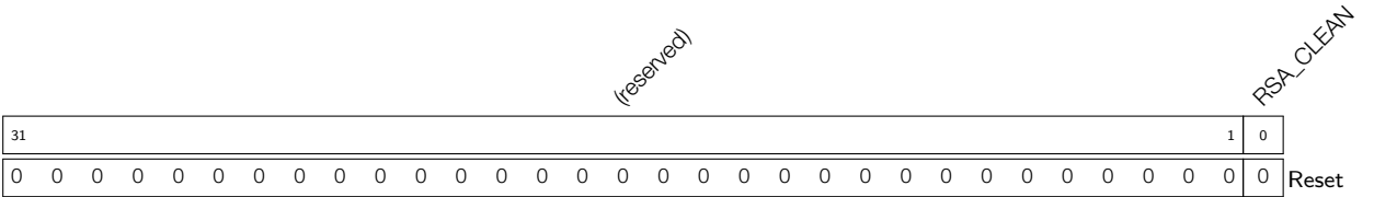
Register 22.7: RSA_CLEAN_REG (0x818)
