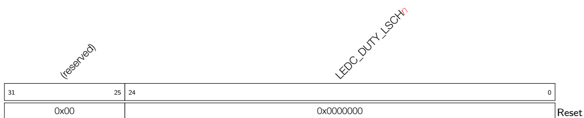
Register 14.8: LEDC_LSCH n _DUTY_REG ( n : 0-7) (0xC4+0x10* n )
