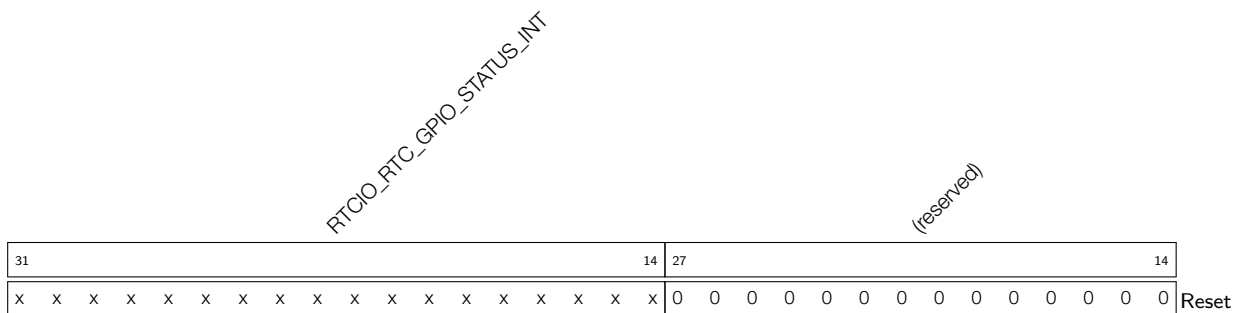
Register 4.41: RTCIO_RTC_GPIO_STATUS_REG (0x0018)
