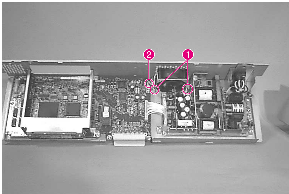
Figure 6-226 Fan
