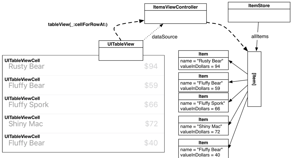
Figure 10.11 UITableViewCell retrieval
