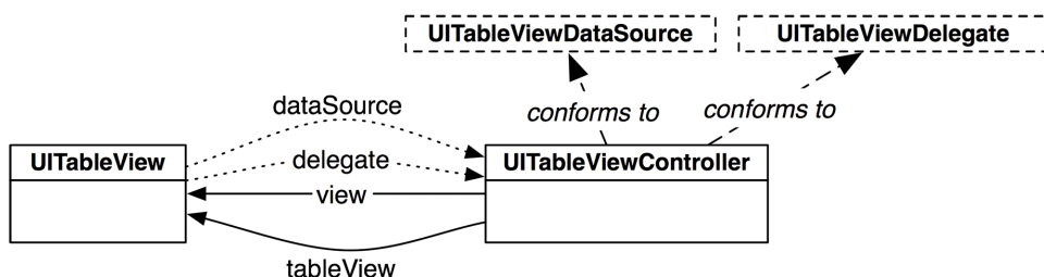
Figure 10.4 UITableViewController-UITableView relationship
