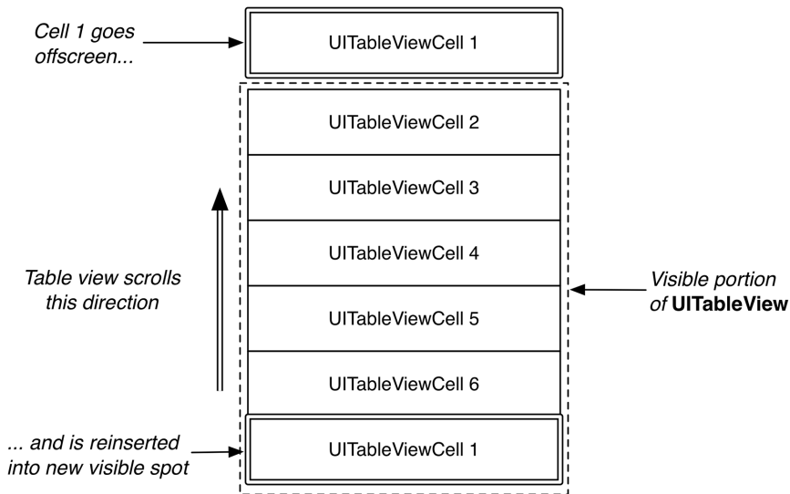
Figure 10.12 Reusable instances of UITableViewCell
