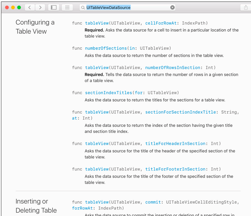
Figure 10.7 UITableViewDataSource protocol documentation
