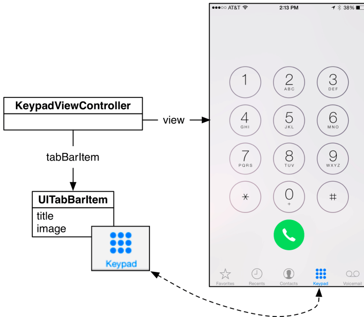
Figure 5.11 UITabBarItem example
