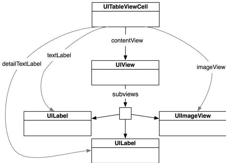
Figure 10.9 UITableViewCell hierarchy
