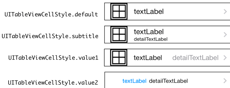
Figure 10.10 UITableViewCellStyle : styles and constants
