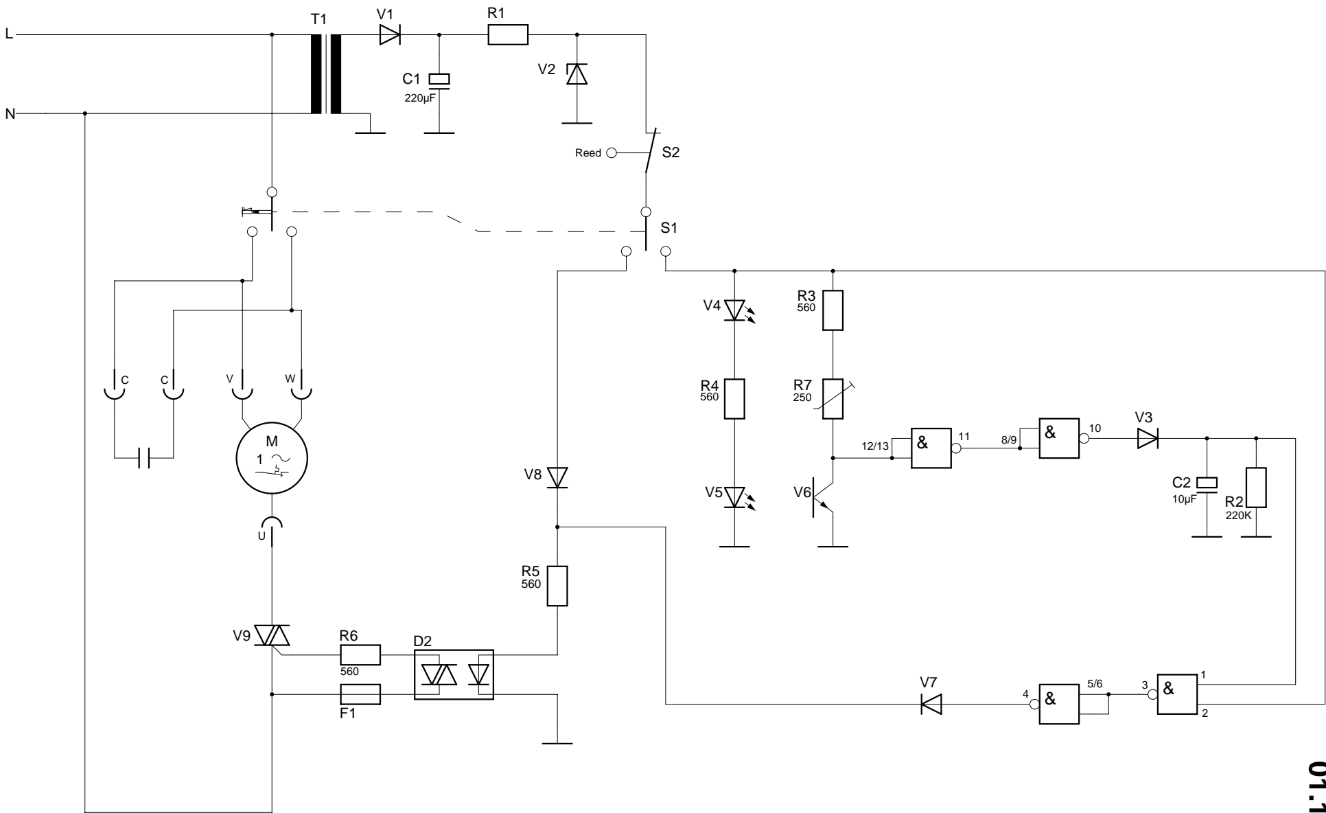
Stromlaufplan 2240 A Cross/Cut schema de circuit électrique 2240 A Cross/Cut wiring diagram 2240 A Cross/Cut
