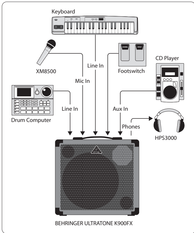
Afb. 3.1: Voorbeeld-setup met de ULTRATONE
