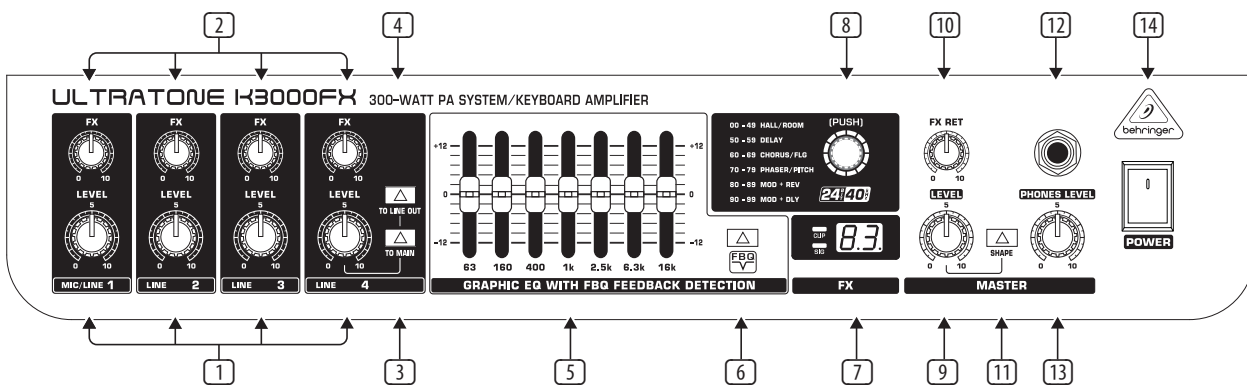
Afb. 2.1: Bedieningselementen op het frontpaneel (K3000FX en K1800FX)
