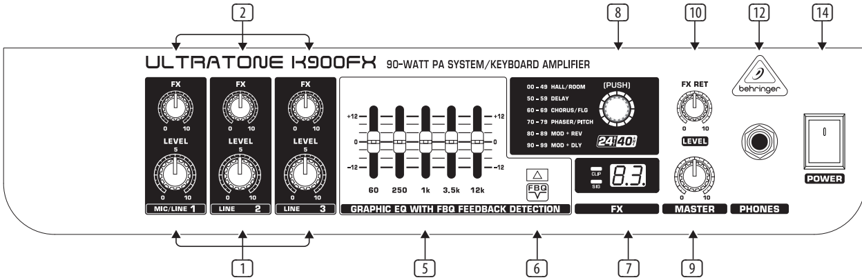
Afb. 2.3: Bedieningselementen op het frontpaneel (K900FX en K450FX)
