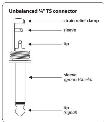
Afb. 4.1: 6,3-mm-monoklinkerstekker
