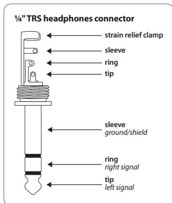
Afb. 4.2: 6,3-mm-stereoklinkerstekker
