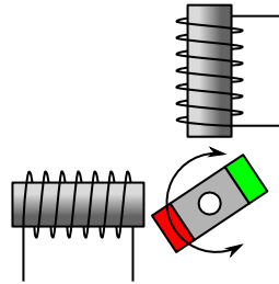
Abbildung 6.12: Vereinfachtes Schema eines Schrittmotors
