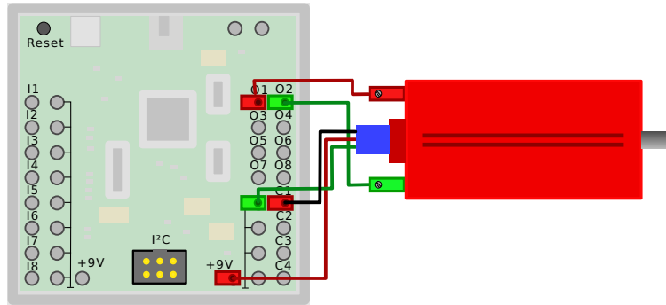
Abbildung 6.8: Anschluss des TXT-Encoder-Motors zur PWM-abhängigen Drehzahlmessung
