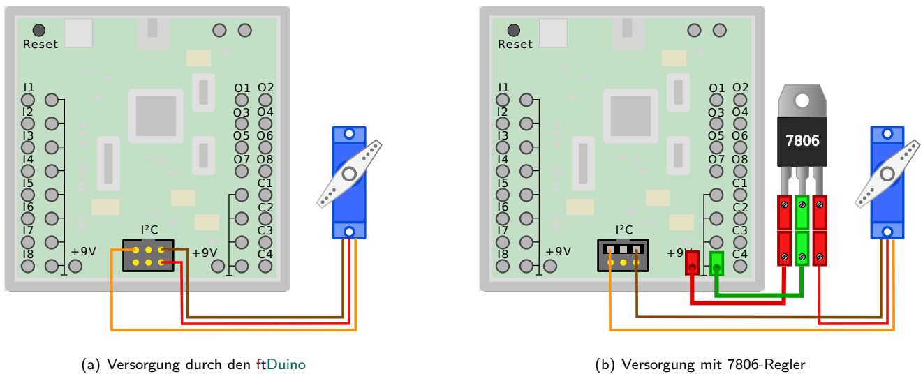
Abbildung 6.15: Anschluss des Servos an den ftDuino
