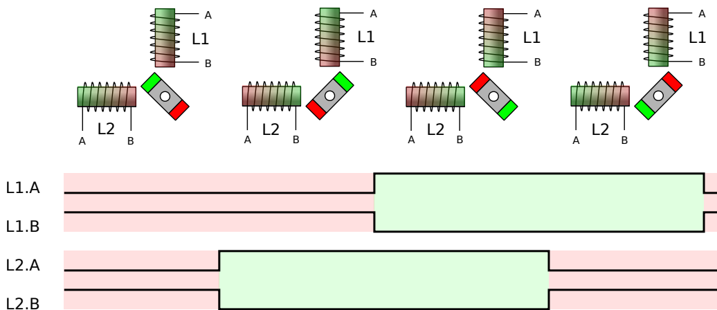
Abbildung 6.13: Vollschrittsteuerung eines Schrittmotors
