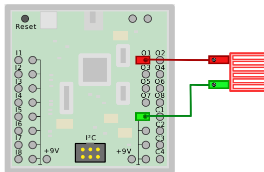
Abbildung 4.8: Lampe an Ausgang O1
