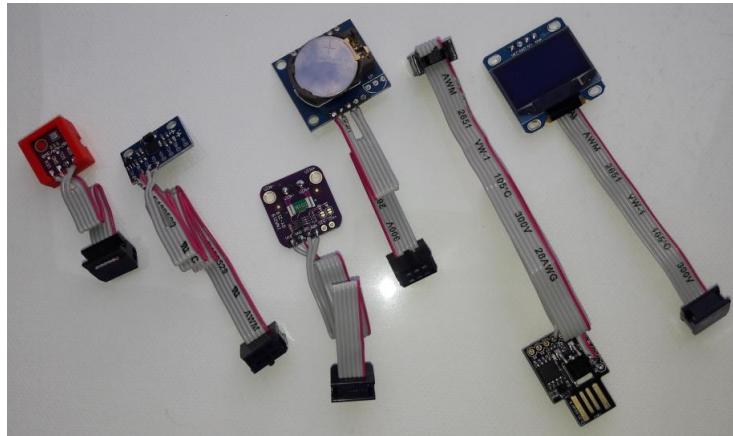
Abbildung 6.31: Diverse I 2 C-Sensoren mit passendem Anschlusskabel an den ftDuino
