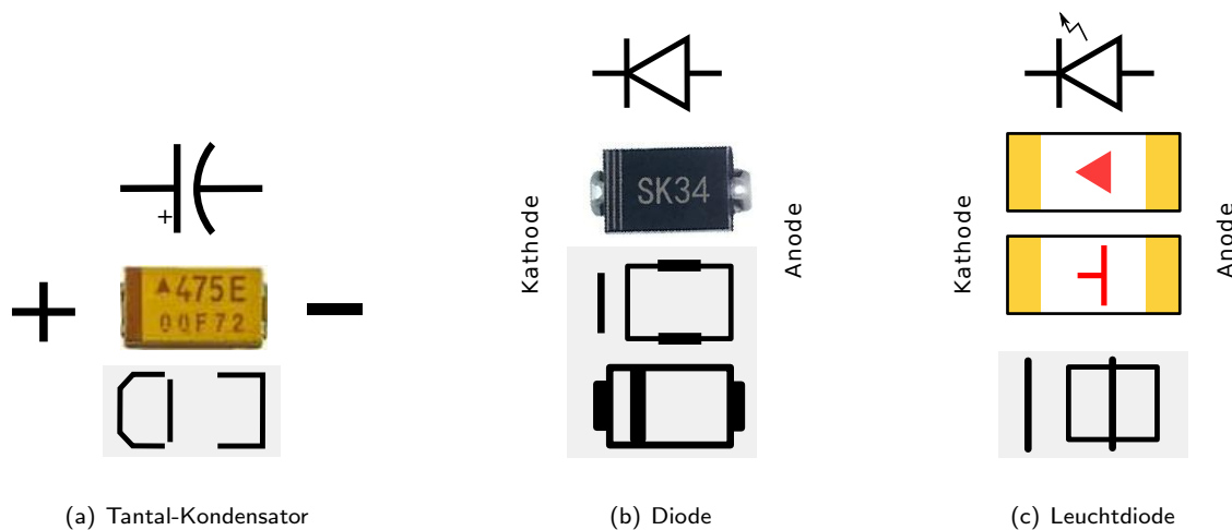
Abbildung 10.2: Schaltplansymbol, Bauteilepolarität und Bestückungssymbol
