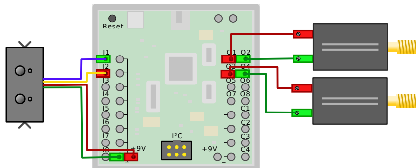
Abbildung 7.5: Verdrahtungsschema des Linienfolgers
