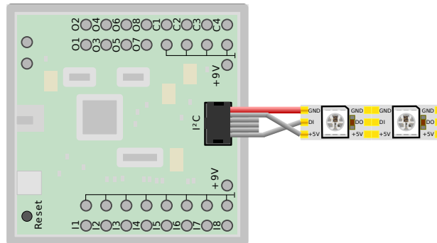
Abbildung 6.49: Anschluss von zwei WS2812B-Vollfarb-Leuchtdioden
