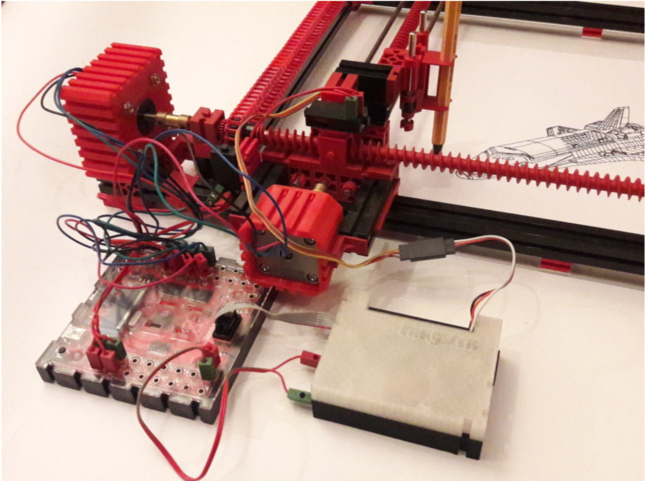
Abbildung 7.8: Der Stift wird von einem fischertechnik-Servo gehoben
