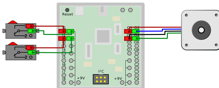
Abbildung 6.11: Anschluss des Schrittmotors an den ftDuino
