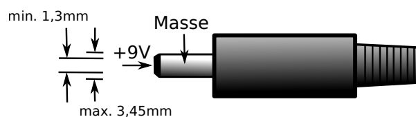
Abbildung 1.8: 3,45mm fischertechnik-Hohlstecker
