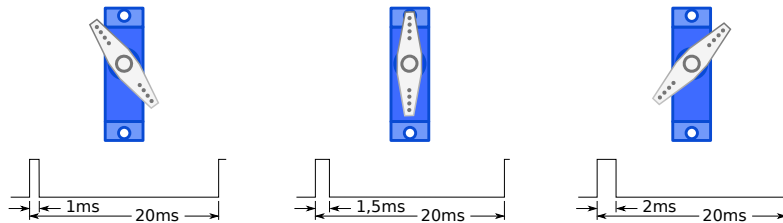
Abbildung 6.17: Servo-Winkel in Abhängigkeit vom Stellsignal
