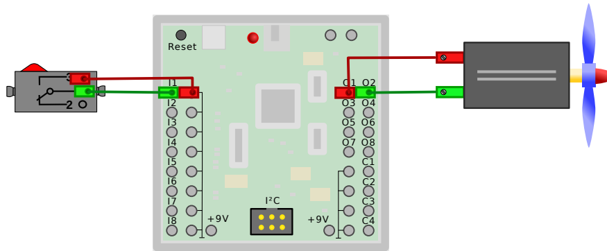
Abbildung 6.2: Not-Aus
