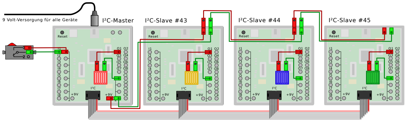
Abbildung 6.38: Kopplung von vier ftDuoinos über I 2 C
