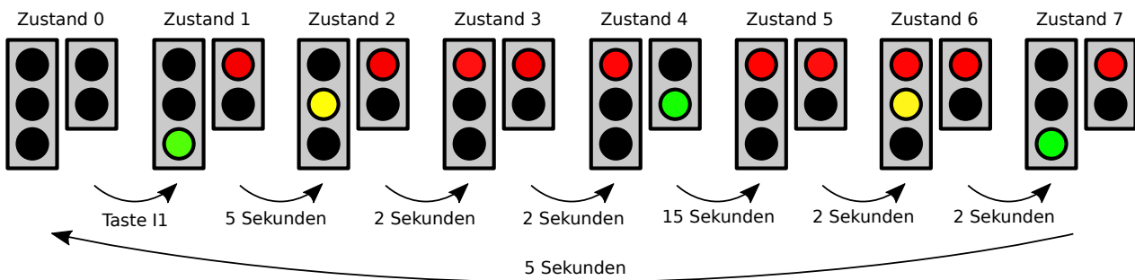
Abbildung 7.7: Die Zustände der Ampel
