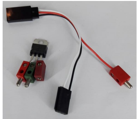
(b) Spannungsregler und Adapterkabel
