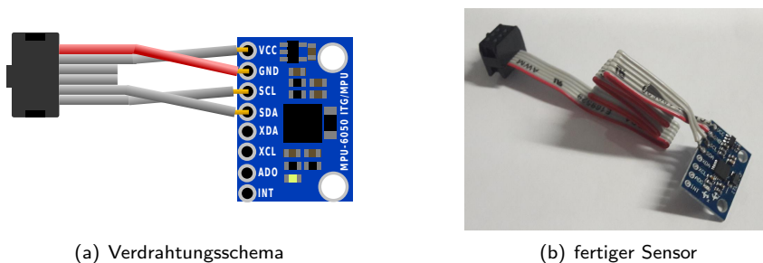
Abbildung 6.30: MPU6050-Sensor mit Anschlusskabel für den ftDuino
