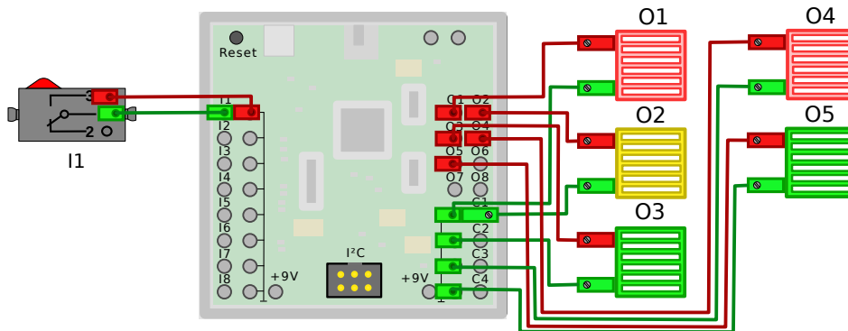
(a) Verdrahtungsschema
