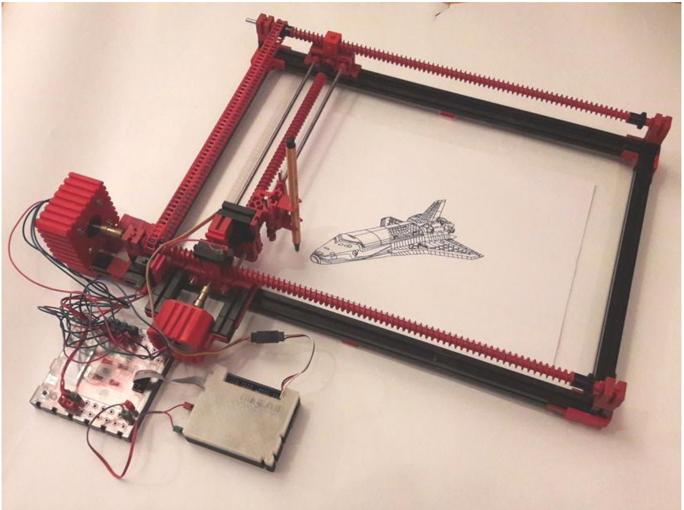
Abbildung 7.9: Das Design orientiert sich stark am Plotter von 1985
