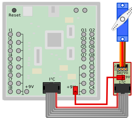
Abbildung 6.48: Anschluss des Mini-I 2 C-Adapters an den ftDuino
