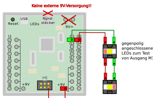
Abbildung 10.7: Testweise Brücke zwischen 5V und 9V
