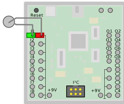
Abbildung 6.20: Anschluss des Temperatursensors an Eingang I1
