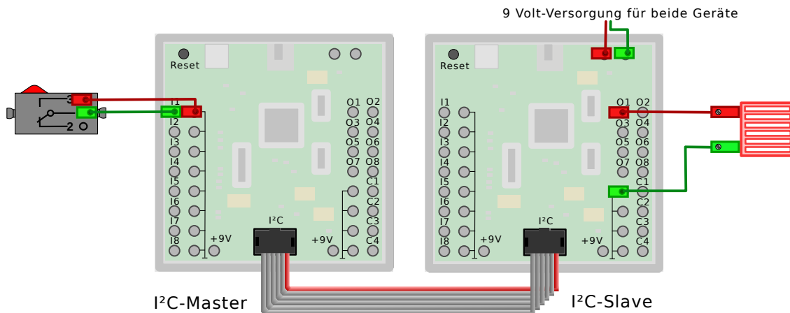
Abbildung 6.37: Kopplung zweier ftDuinos über I 2 C
