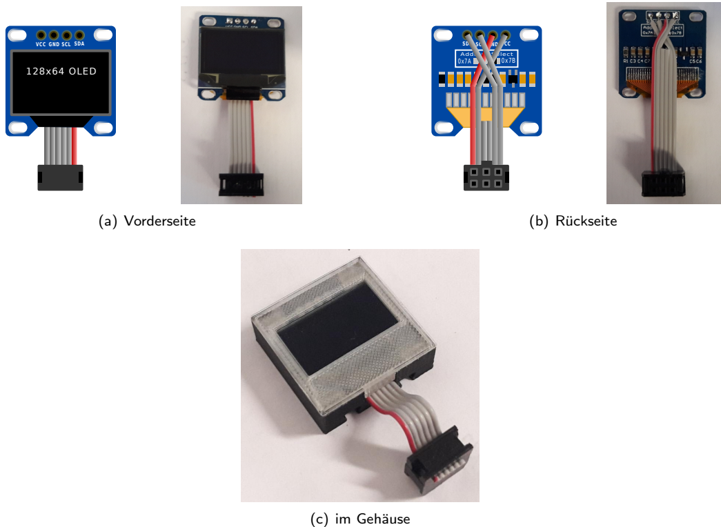
Abbildung 6.34: OLED-Display mit Anschlusskabel für den ftDuino
