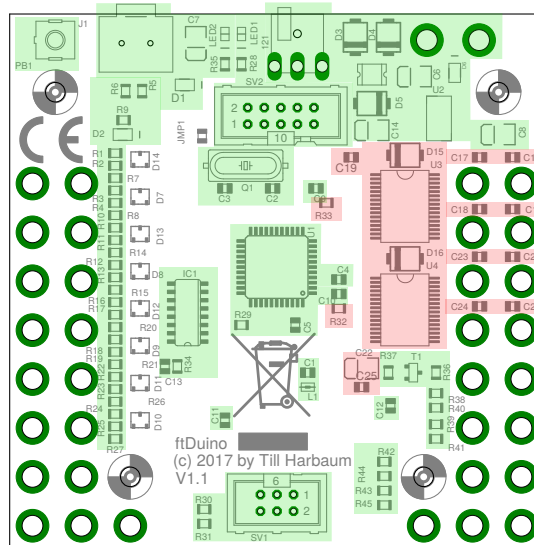
Abbildung 10.6: Komponenten der Ausgänge
