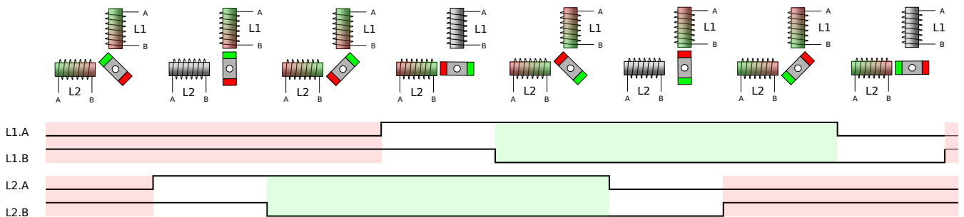
Abbildung 6.14: Halbschrittsteuerung eines Schrittmotors
