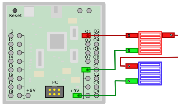
Abbildung 6.21: Zwei Lampen an Ausgang 01
