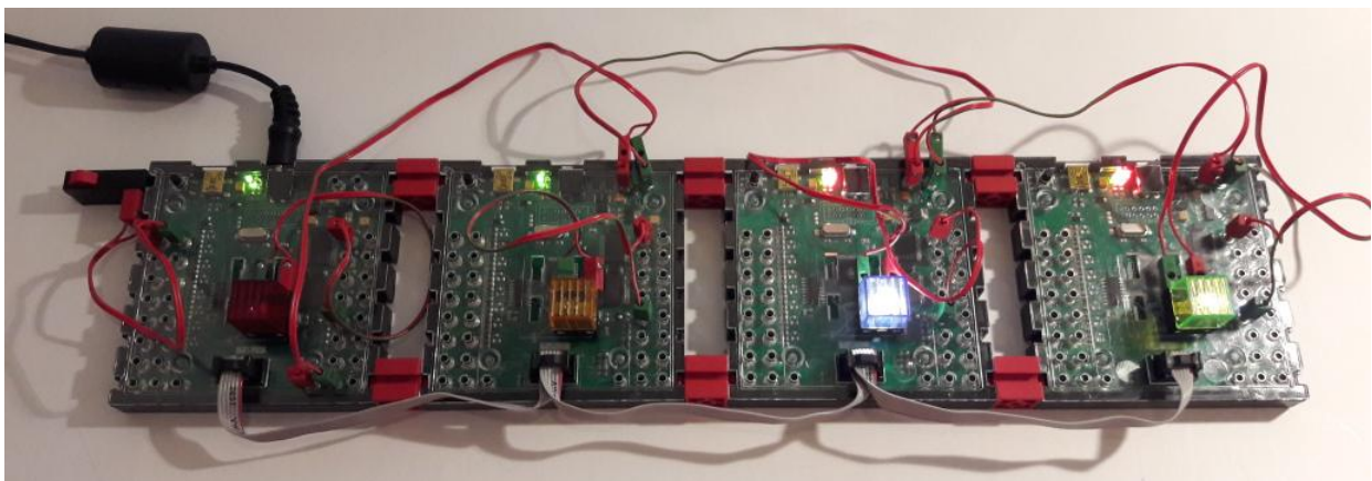
Abbildung 6.39: Vier ftDuoinos über I 2 Cgekoppelt
