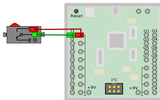
Abbildung 6.28: Entprellen
