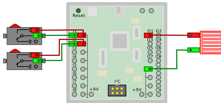
Abbildung 6.5: Pulsweitenmodulation
