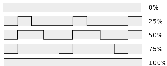
Abbildung 6.7: Ausgewählte PWM-Verhältnisse von 0 bis 100%
