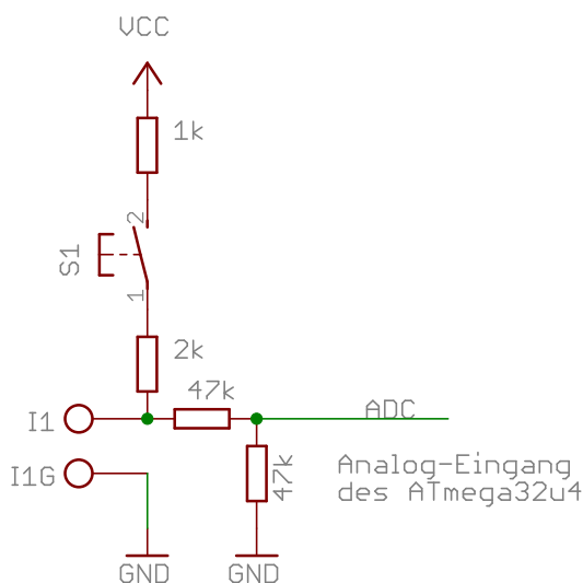
Abbildung 6.18: Interne Beschaltung der Eingänge I1 bis I8 des ftDuino
