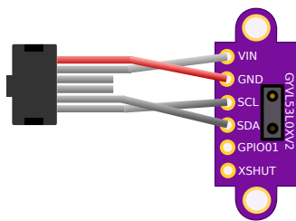
Abbildung 6.35: Anschlussschema des VL53L0X an den ftDuino
