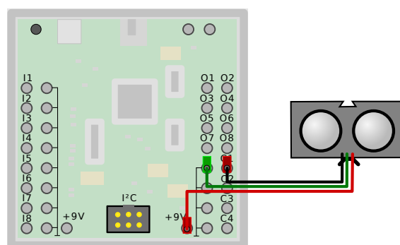
Abbildung 1.12: Anschluss des Ultraschallsensors 133009
