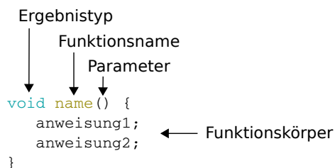
Abbildung 4.6: Funktionsdefinition
