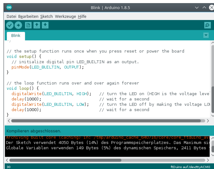
Abbildung 5.12: Die Arduino-IDE
