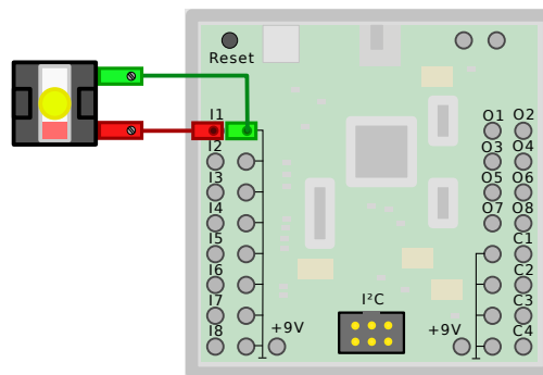
Abbildung 6.19: Anschluss einer LED an Eingang I1 des ftduino
