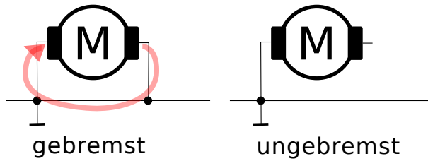
Abbildung 6.23: Elektrisch gebremster und ungebremster Elektromotor
