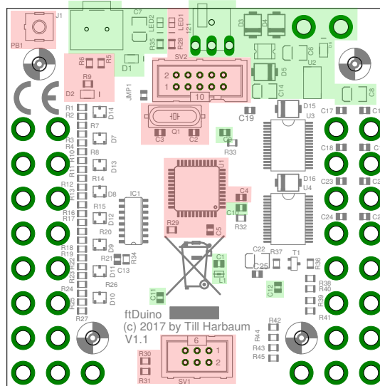
Abbildung 10.3: Komponenten des Mikrocontrollers
