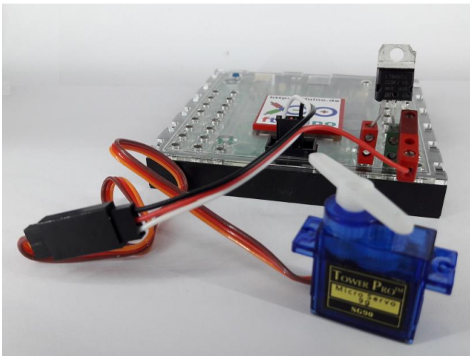
(a) Servo an Regler und Adapterkabel
