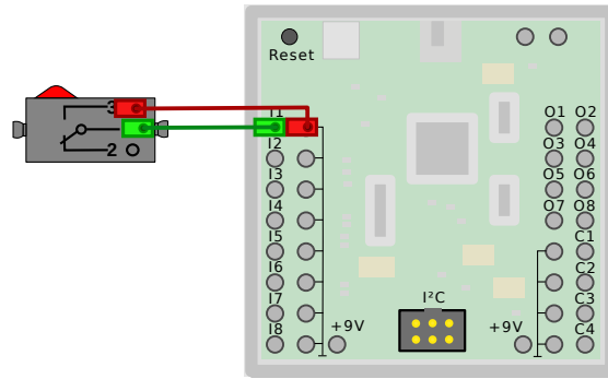
Abbildung 4.10: Taster an Eingang I1
