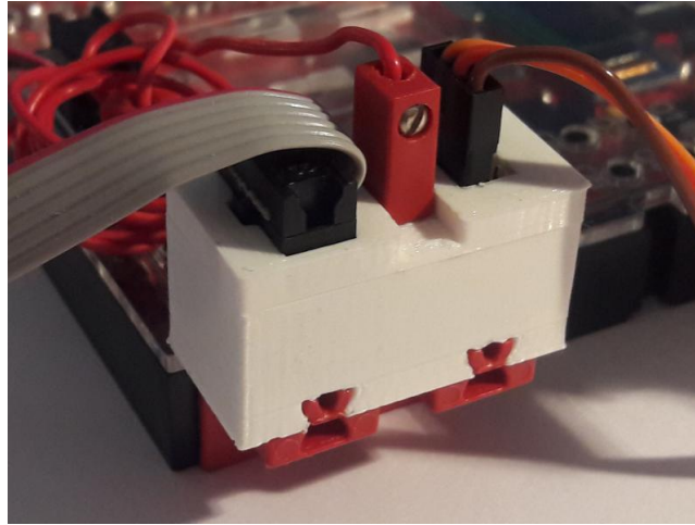
Abbildung 6.47: Der Mini-I 2 C-Adapter am ftDuino
