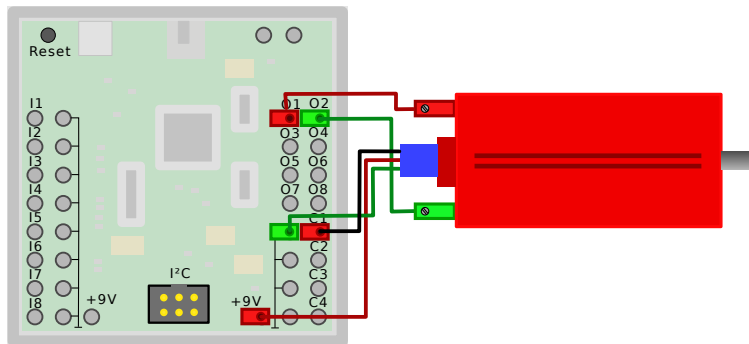
Abbildung 6.24: Anschluss des TXT-Encoder-Motors an die Anschlüsse M1 und C1
