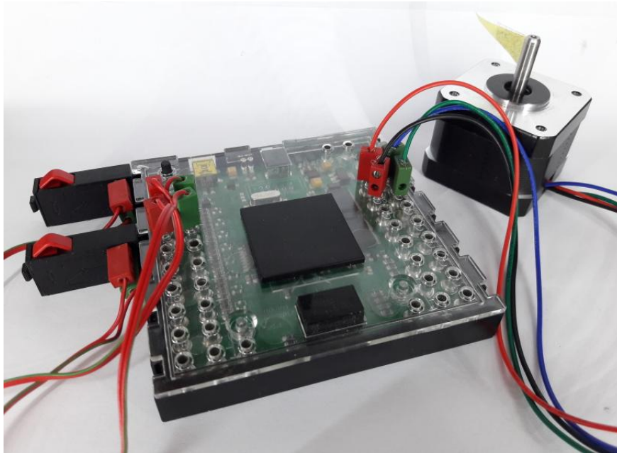
Abbildung 6.10: 17HS13-Schrittmotor am ftDuino
