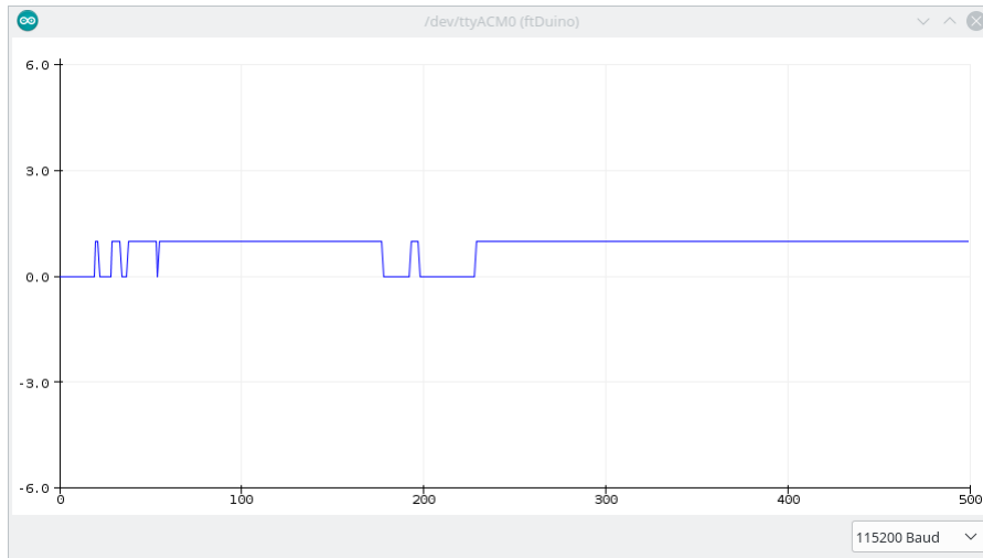
Abbildung 6.29: Verlauf des Prellens im seriellen Plotter
