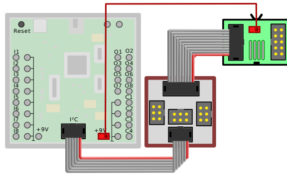
Abbildung 6.43: Anschluss eines fischertechnik-Sensors via I 2 C-Expander
