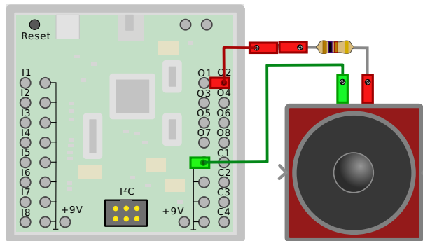
Abbildung 6.50: Anschluss der Lautsprecherkassette an den ftDuino
