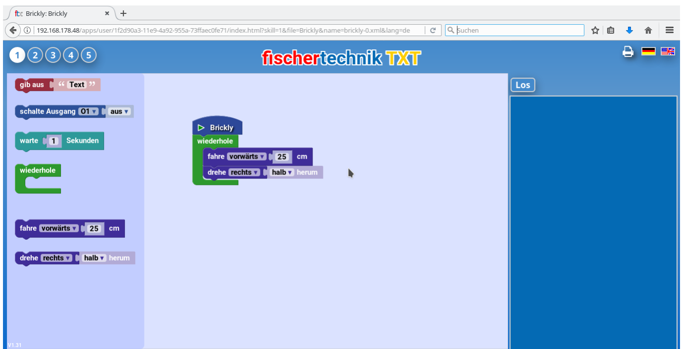
Abbildung 5.9: Die Brickly-Benutzeroberfläche
