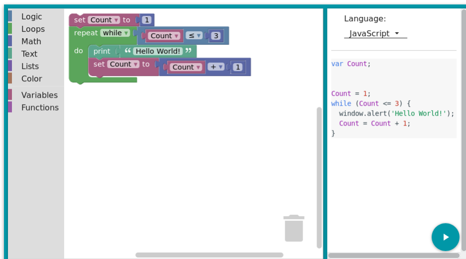
Abbildung 5.8: Die Blockly-Benutzeroberfläche
