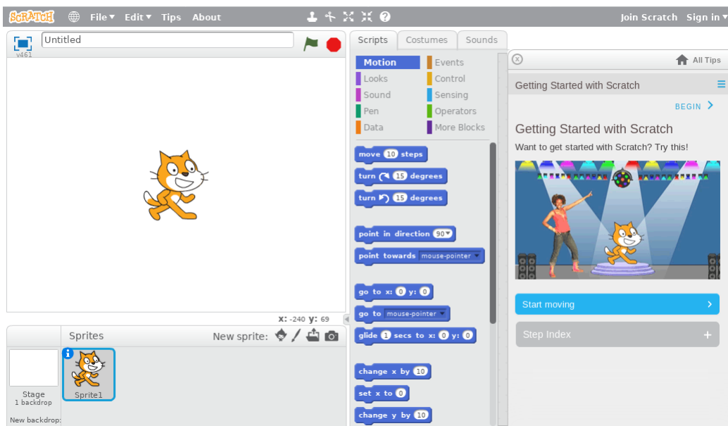
Abbildung 5.2: Die Scratch-2.0-Programmierungsumgebung
