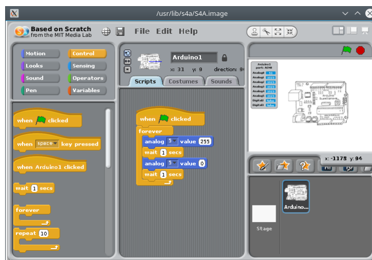
Abbildung 8.9: S4A-Hauptbildschirm
