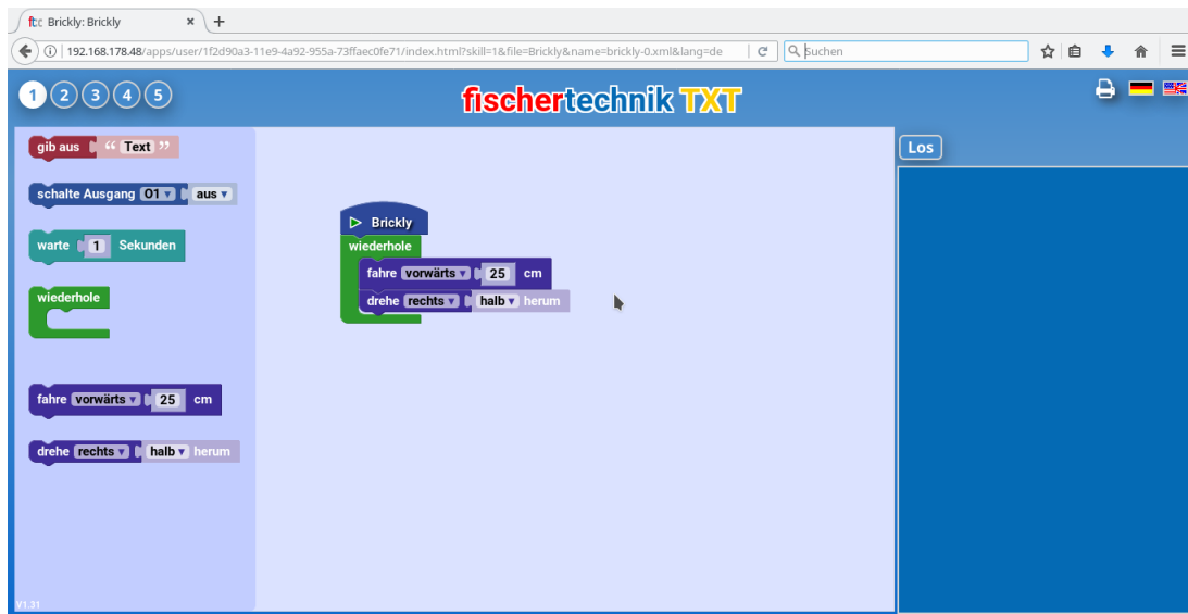
Abbildung 8.4: Die Brickly-Programmiersoberfläche
