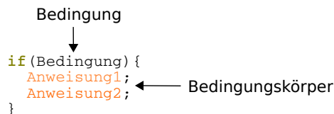
Abbildung 4.9: if-Anweisung
