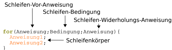
Abbildung 4.12: for -Schleife
