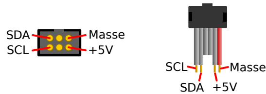
Abbildung 1.13: Buchsen- und Kabelbelegung des I 2 C-Bus am ftDuino
