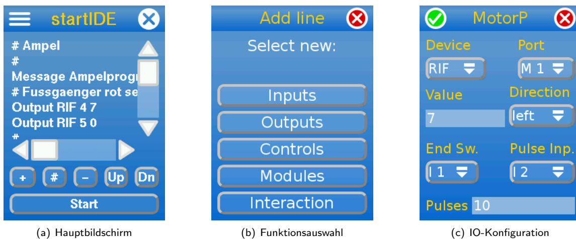
Abbildung 8.7: Die Oberfläche der StartIDE
