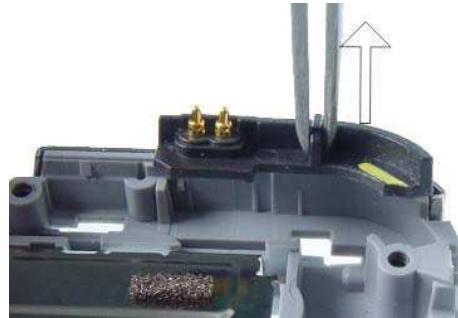
27.) Remove the Bluetooth Antenna .
