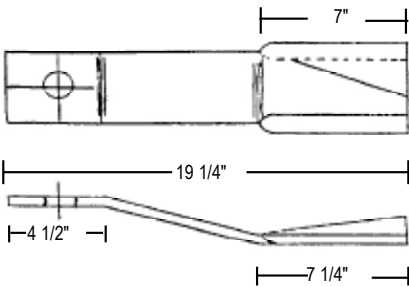
Catalog No. 125-1205
