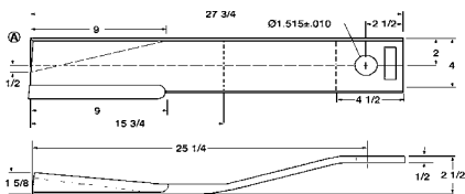
Catalog No. 800-7556
