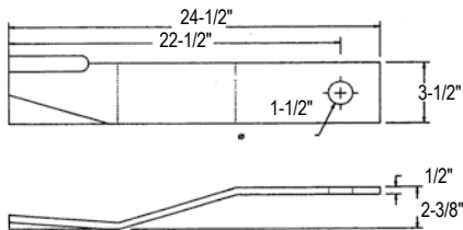
Catalog No. 125-1415
