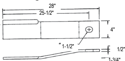
Catalog No. 401-032
