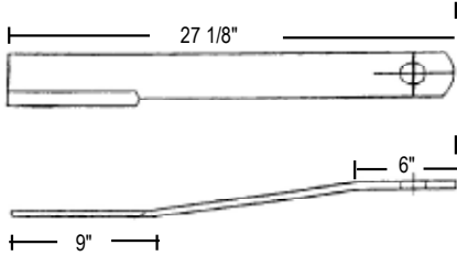
Catalog No. 125-1102
