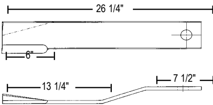
Catalog No. 125-1371
