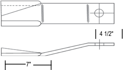
Catalog No. 125-1205
