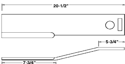
Catalog No. 125-1406
