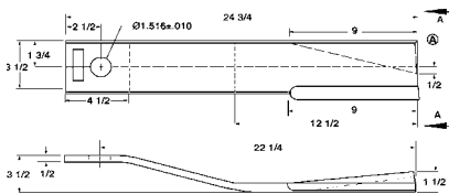
Catalog No. 125-1454
