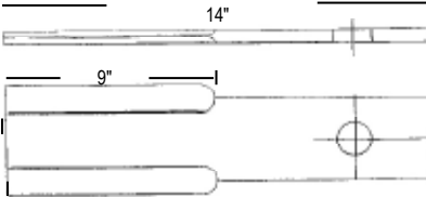
Catalog No. 125-1451
