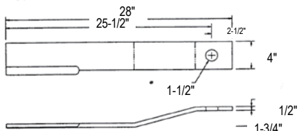
Catalog No. 401-028
