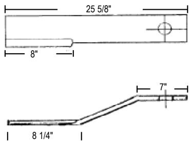
Catalog No. 125-1404
