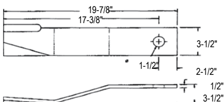
Catalog No. 00753841
