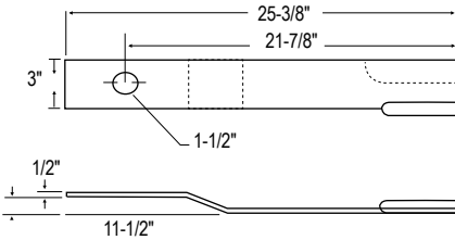
Catalog No. 125-1152
