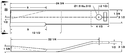
Catalog No. 125-1453
