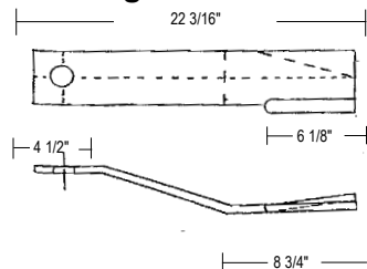
Catalog No. 125-1366
