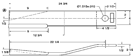
Catalog No. 800-7555
