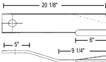
Catalog No. 125-1401
