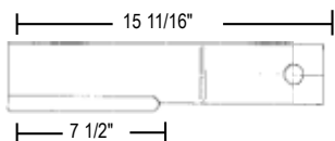
Catalog No. 125-1360
