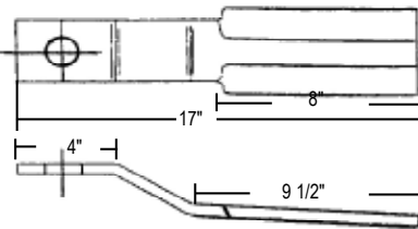
Catalog No. 125-1302
