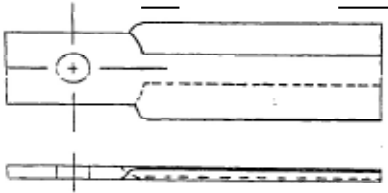
Catalog No. 125-1301
