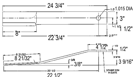
Catalog No. 125-1362
