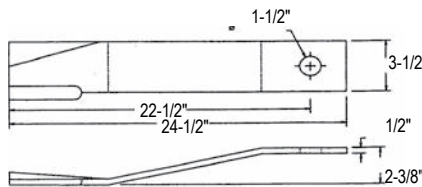
Catalog No. 125-1416
