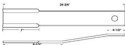
Catalog No. 125-1361
