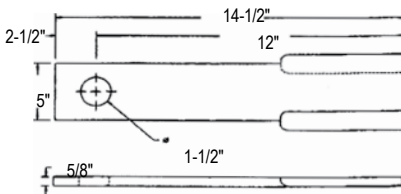
Catalog No. 125-1455
