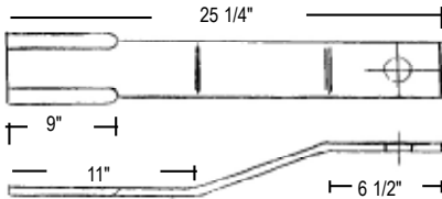
Catalog No. 125-1452
