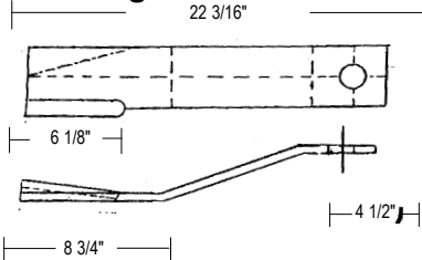
Catalog No. 125-1367
