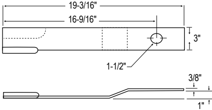
Catalog No. 125-1152
