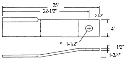
Catalog No. 401-027
