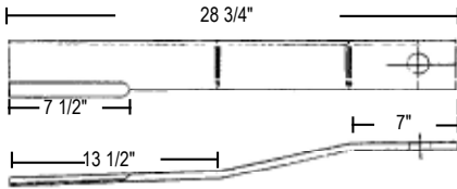
Catalog No. 125-1403
