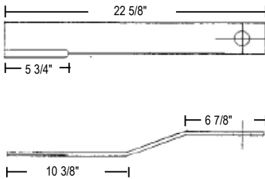
Catalog No. 125-1403
