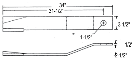
Catalog No. 125-1417
