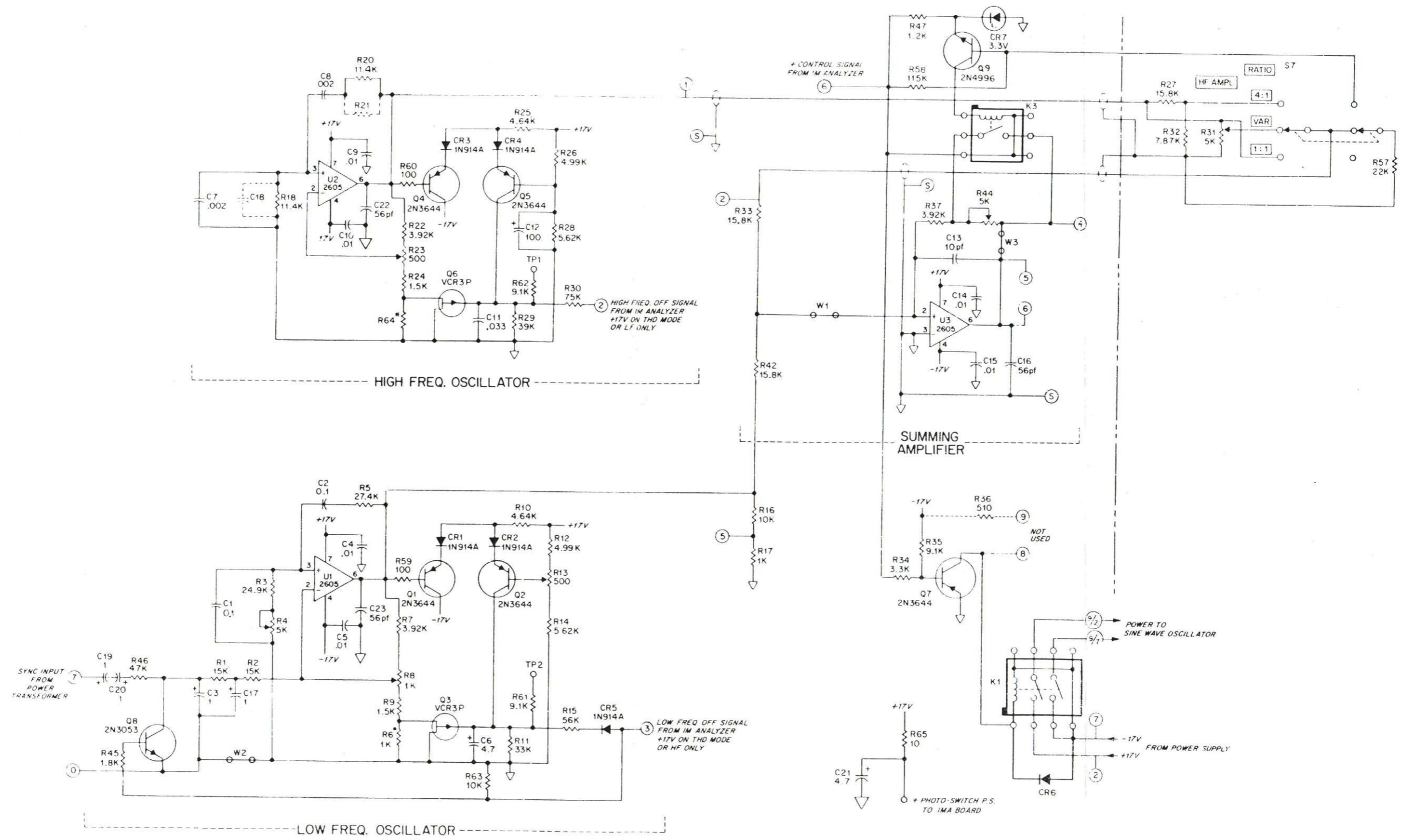
IM GENERATOR
