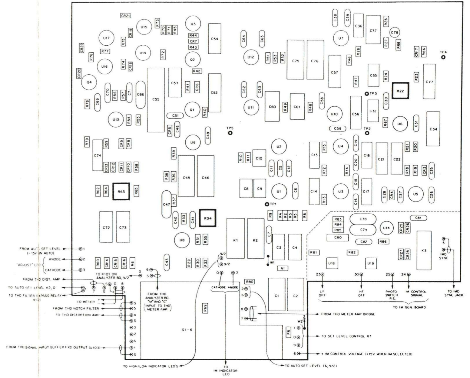
IM ANALYZER
