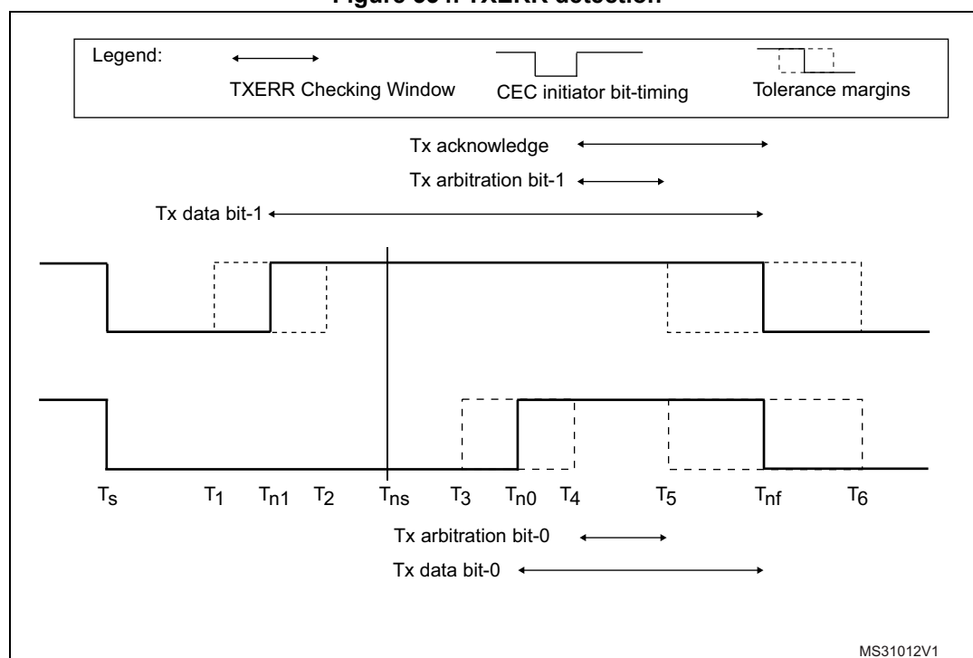
Figure 334. TXERR detection
