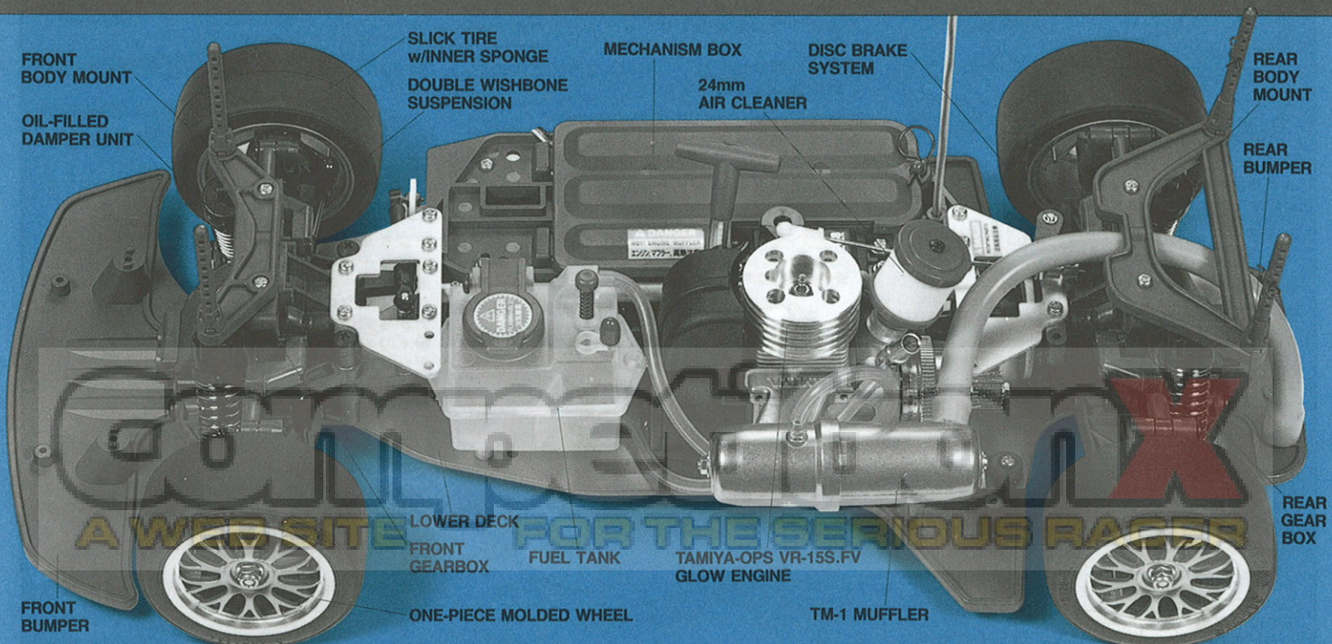
1/8エンジンRC 4WDレーシングカー カルソニック・スカイラインGT-R (TGX-Mk1タミヤ掛川サーキットオープン記念スペシャル)
