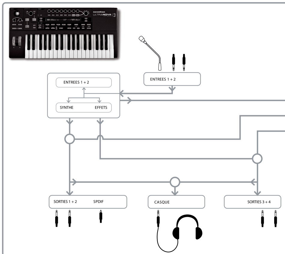
ROUTAGE AUDIO DANS L'ULTRANOVA
