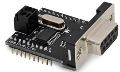
Figure: RS-485/Modbus module
