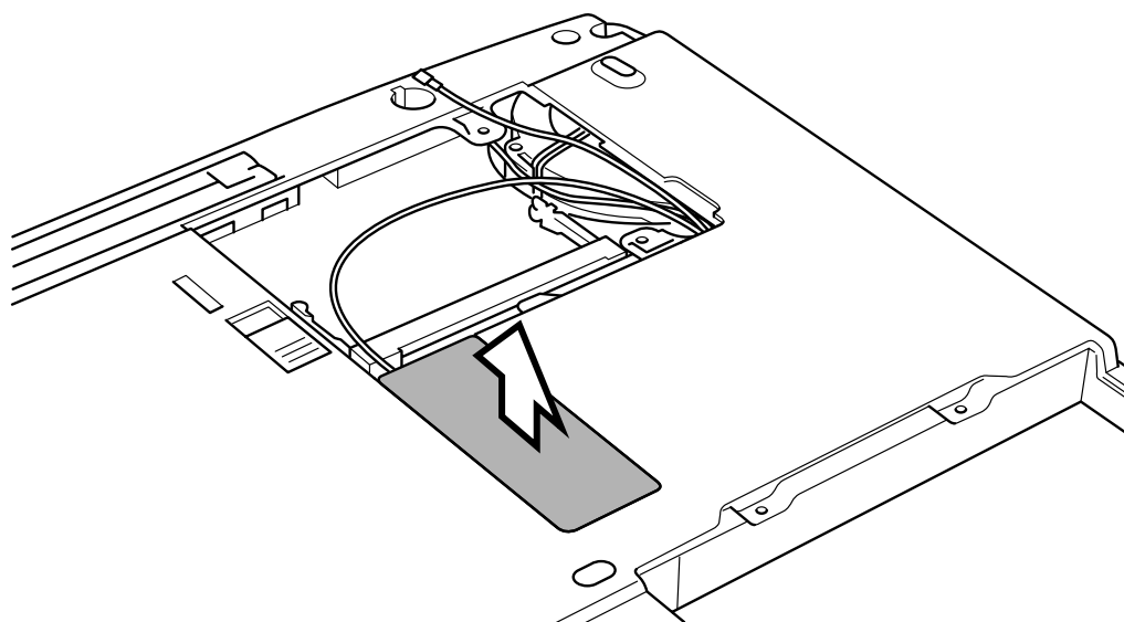
Rimozione del coperchio dello slot per il modulo Bluetooth
