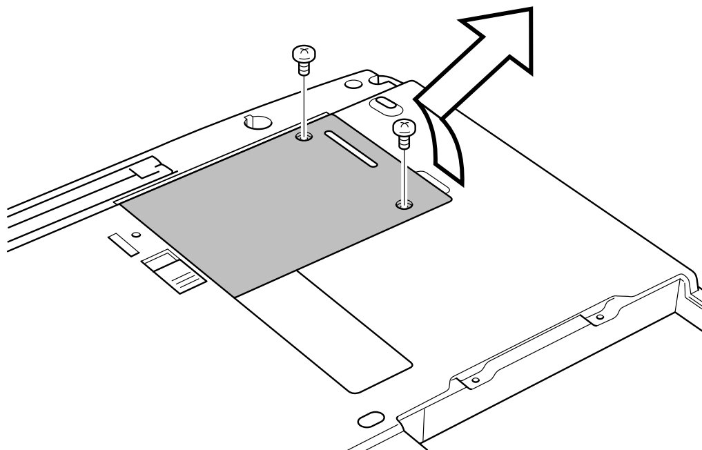
Løfte spordekkelet for Bluetooth-modulen
