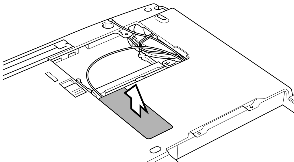
Fjerne spordekkelet for Bluetooth-modulen
