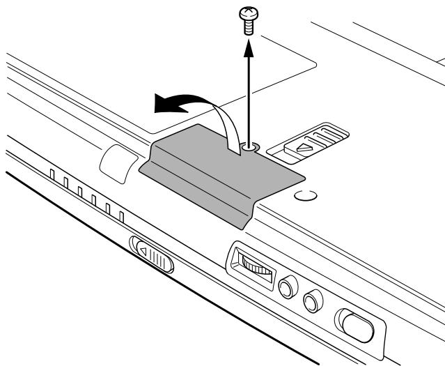
Fjerne spordekkelet for Bluetooth-modulen
