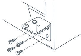
Dibujo 2 Quitar puerta y bisagras
