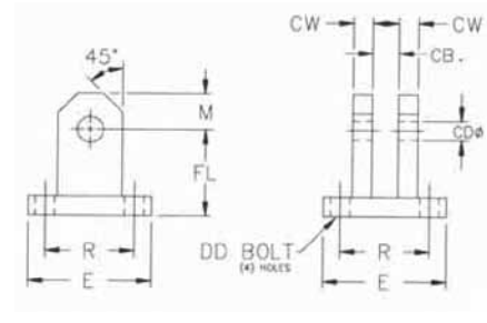
Detachable Clevis
