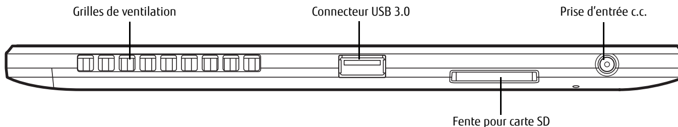
Figure 4. Caractéristiques de la Tablette Hybride STYLISTIC Q704 (vue de gauche)
