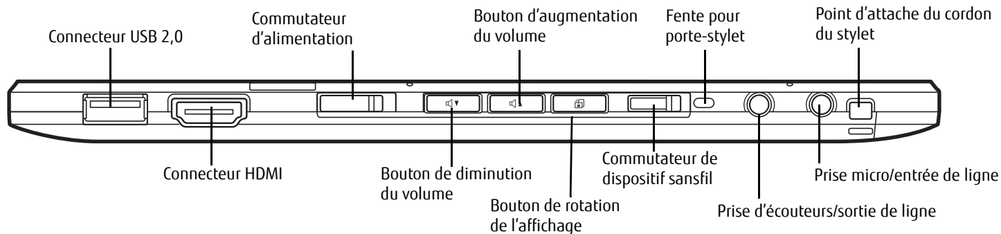
Figure 5. Caractéristiques de la Tablette Hybride STYLISTIC Q702 (vue de droite)
