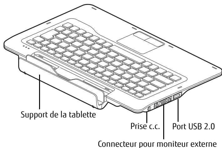
Figure 20. Station d'arrimage - arrière
