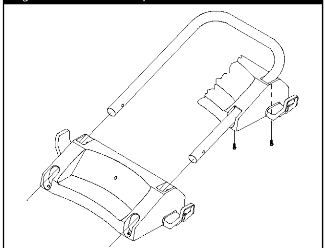
Figura 23 - Conecte Bandeja Accesoría
