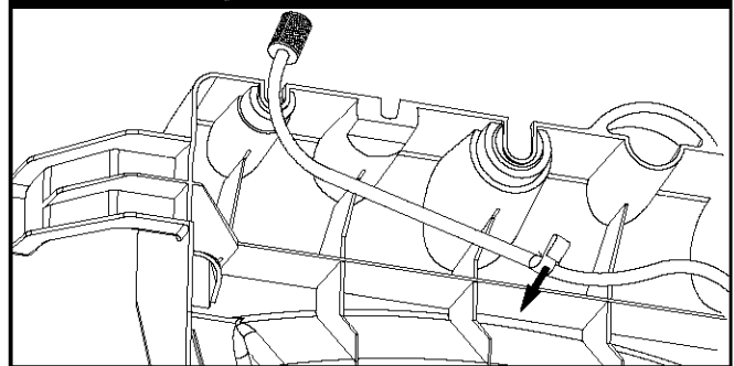
Figure 28 — Deslice Clip de Metal en la Bandeja Accesoria Flange
