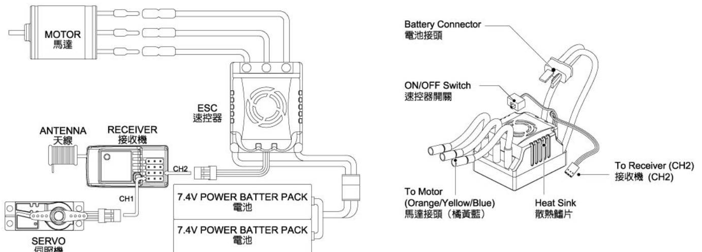
4.2 MODEL WIRING DIAGRAM 電控系統連結圖
