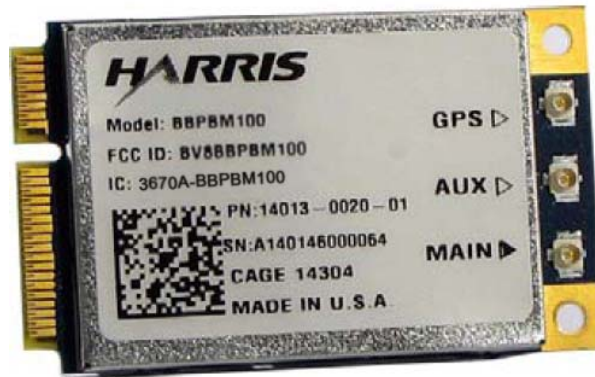
Figure 1-1: PCI Express Mini (PEM) Module
