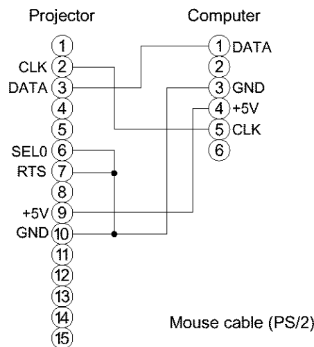
Mouse jack Mini DIN 6-pin
