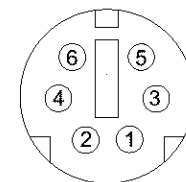
Mouse jack Mini DIN 6-pin
