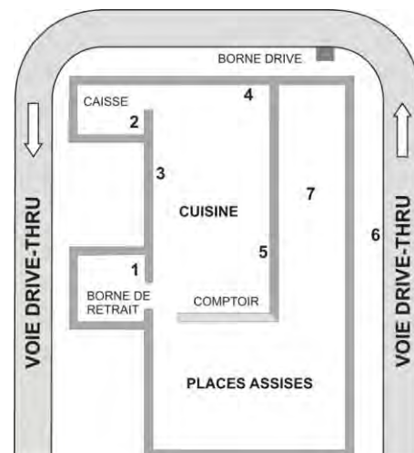
Figure 10. Agencement-type d'un magasin drive-thru
