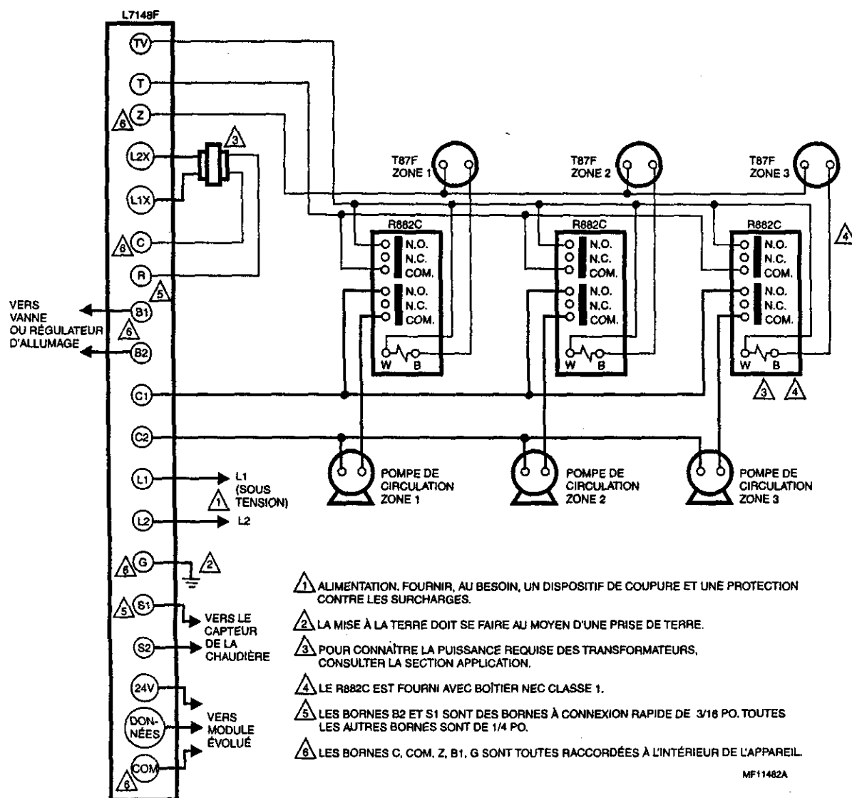
Fig. 8. Système multizone avec pompe de circulation dérivée R882C.
