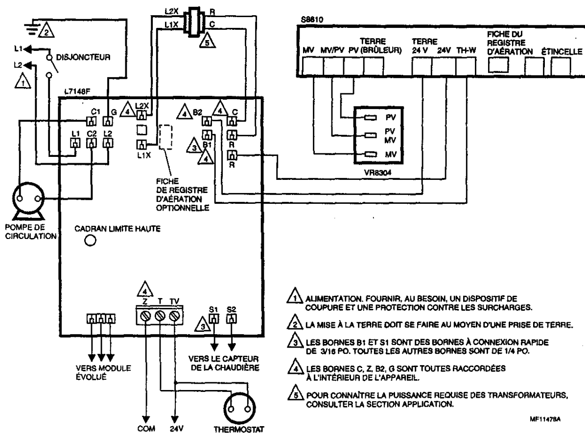
Fig. 6. Raccordement du L7148F avec module d'allumage à veilleuse intermittente S8610 avec fiche pour registre d'aération automatique et registre d'aération D892/D896/M892/M896 de Honeywell.
