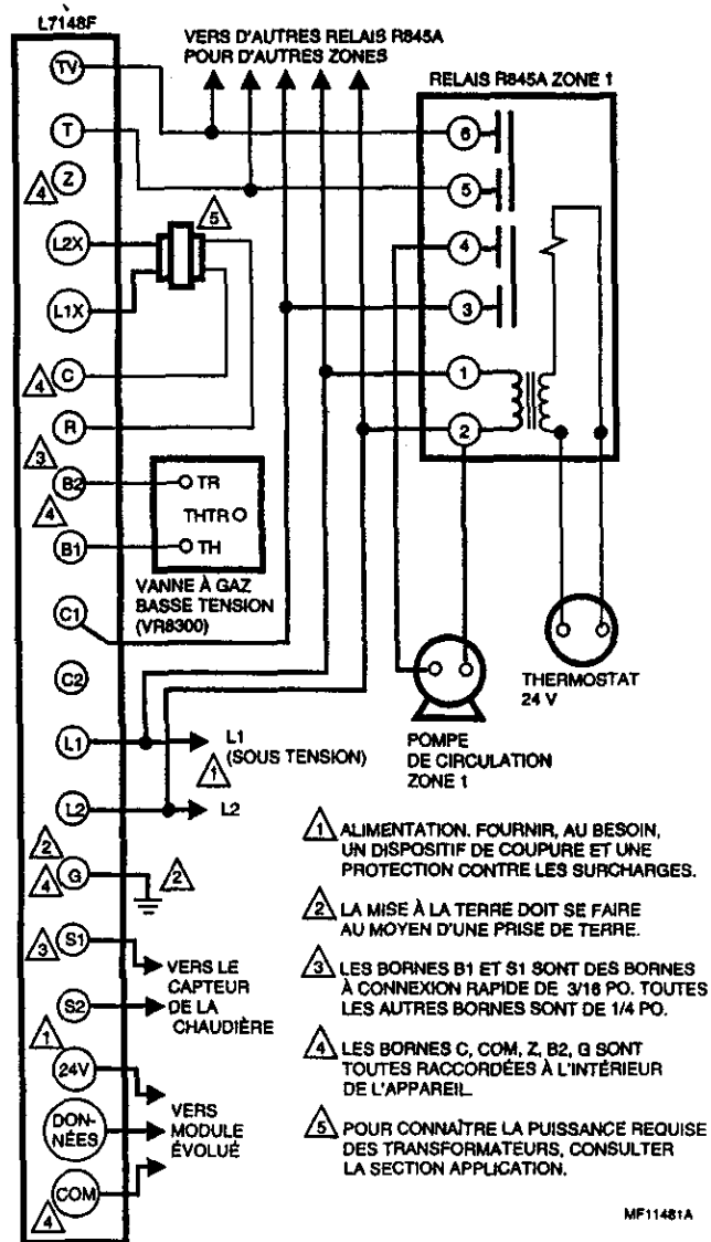
Fig. 5. Raccordement du L7148F dans un système multizone avec pompe de circulation dérivée.
