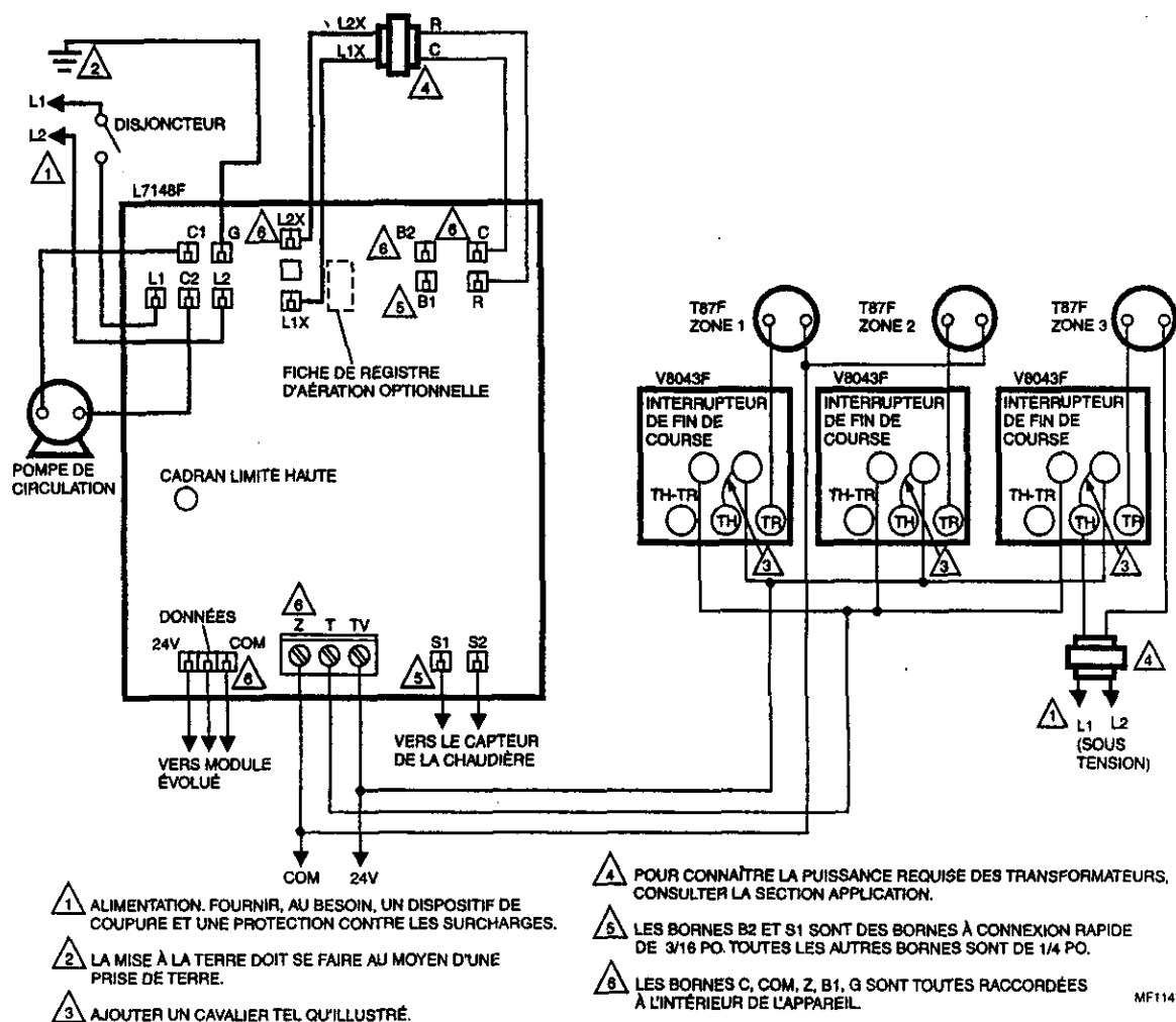
Fig. 3. Raccordement du L7148F à des vannes multizones.
