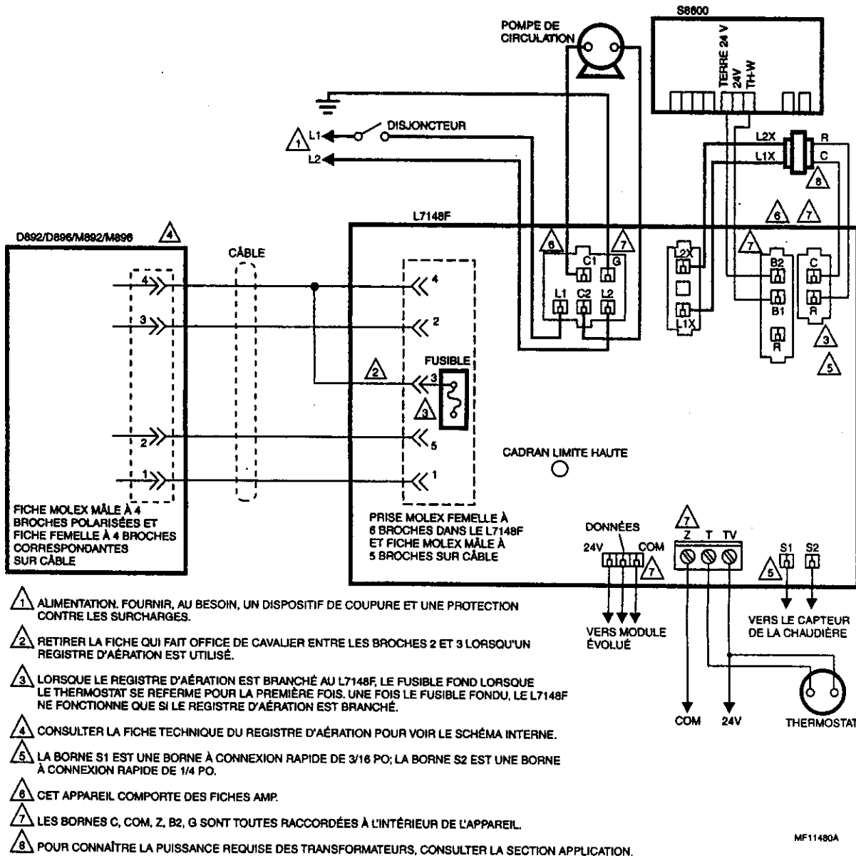
Fig. 7. Raccordement du L7148F avec fiches de raccordement AMP® et raccordement interne direct à un registre d'aération D892/D896/M892/M896 dans un système à eau chaude à veilleuse intermittente.
