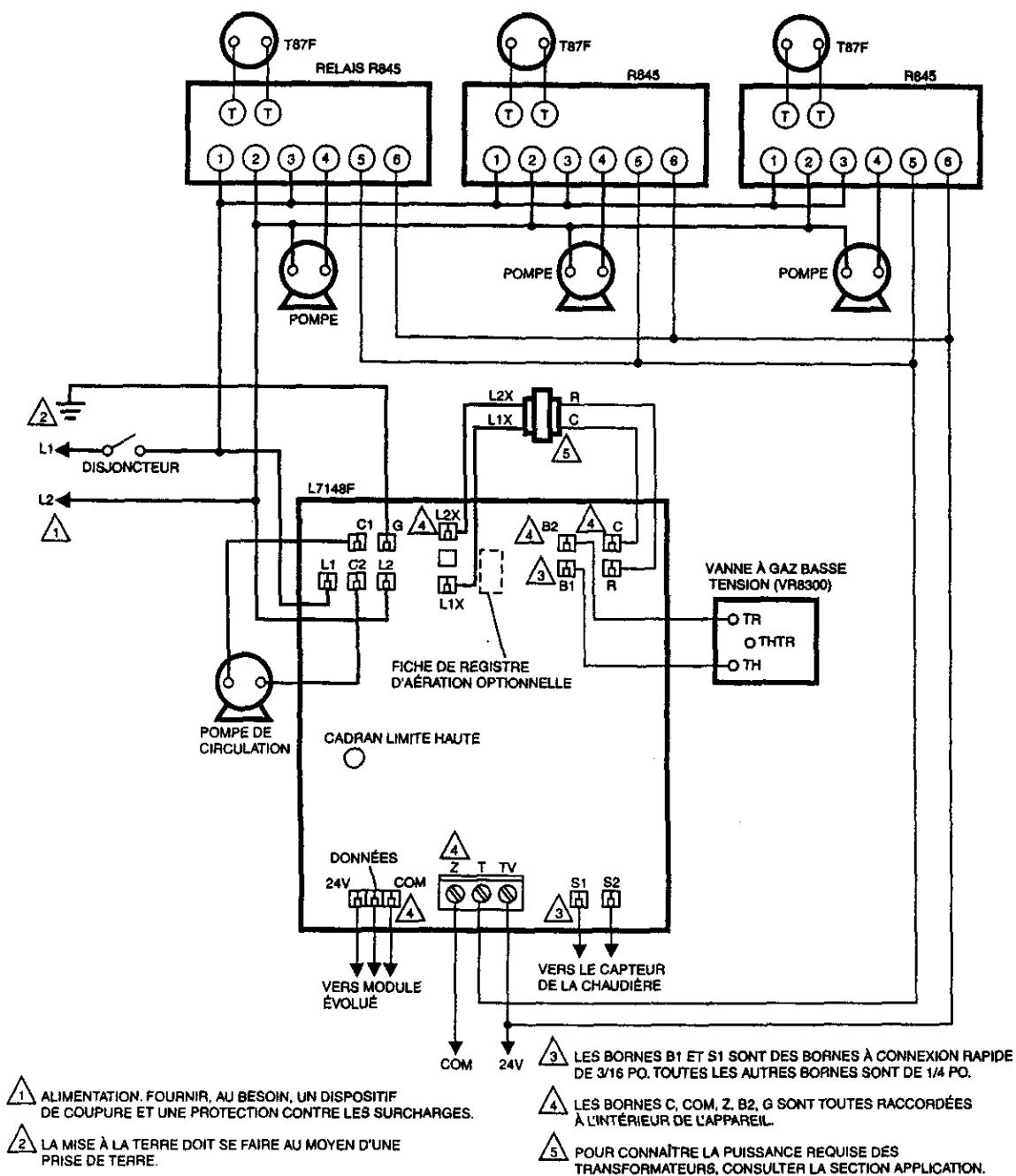
Fig. 4. Raccordement du L7148F dans un système à gaz à circulation forcée d'eau chaude, avec pompe.
