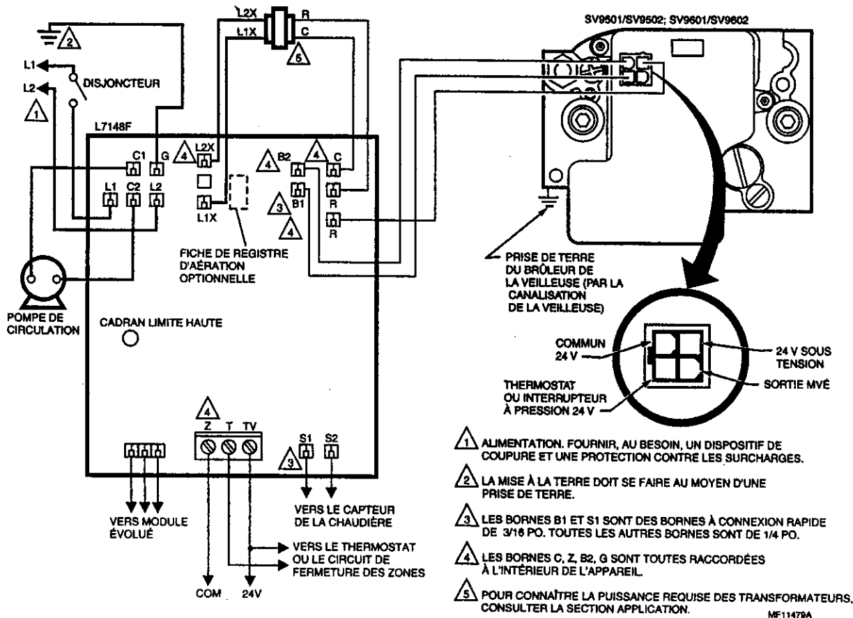
Fig. 9. Raccordement du L7148F à un système de régulation SmartValveMC SV9501/SV9502/SV9601/SV9602.
