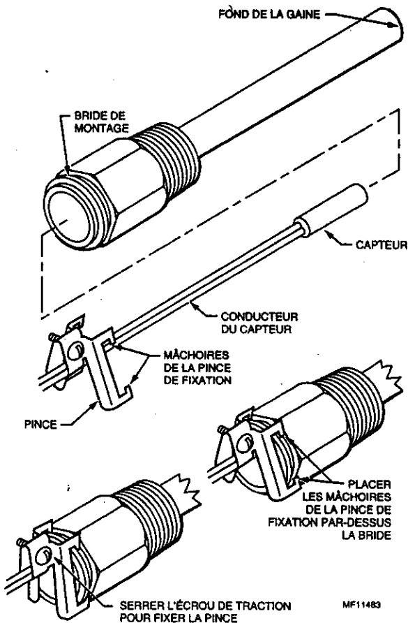
Fig. 1. Fixer le capteur et le conducteur à l'aide de la pince de fixation.
