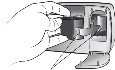
Bakreni kontakti
