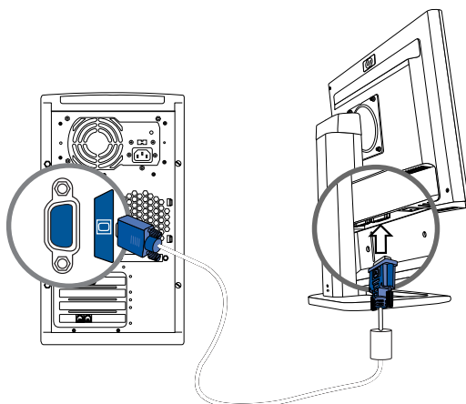
Ligação do cabo de sinal VGA
