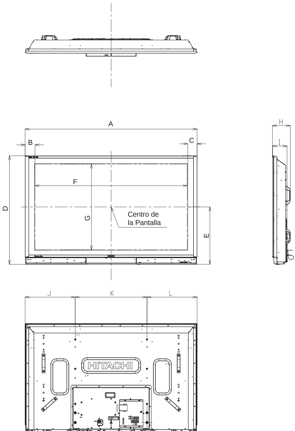
Vista Posterior, úsele como referencia para la instalación en muro.
