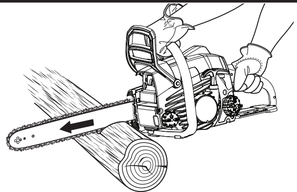
COUPE PAR LE DESSUS
