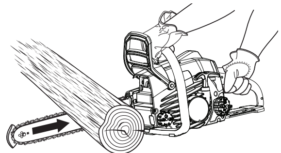
COUPE PAR LE DESSOUS
