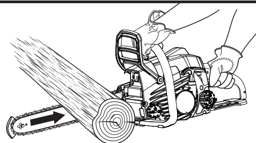
TRONZADO POR ABAJO
