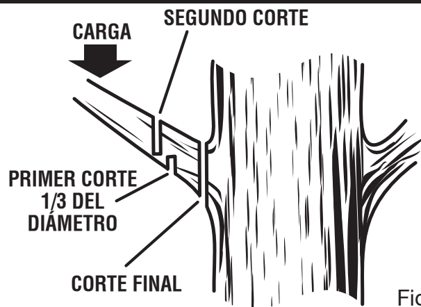
TRONZADO POR ABAJO
